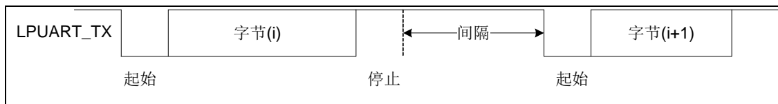
图 5-25 LPUART 发送间隔
