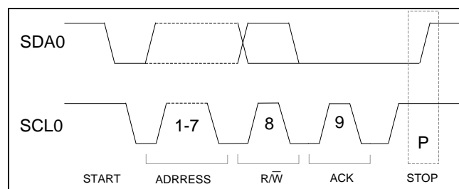
图 5-60 I2C 停止位波形图
