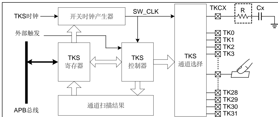
图 5-70 TKS 结构框图
