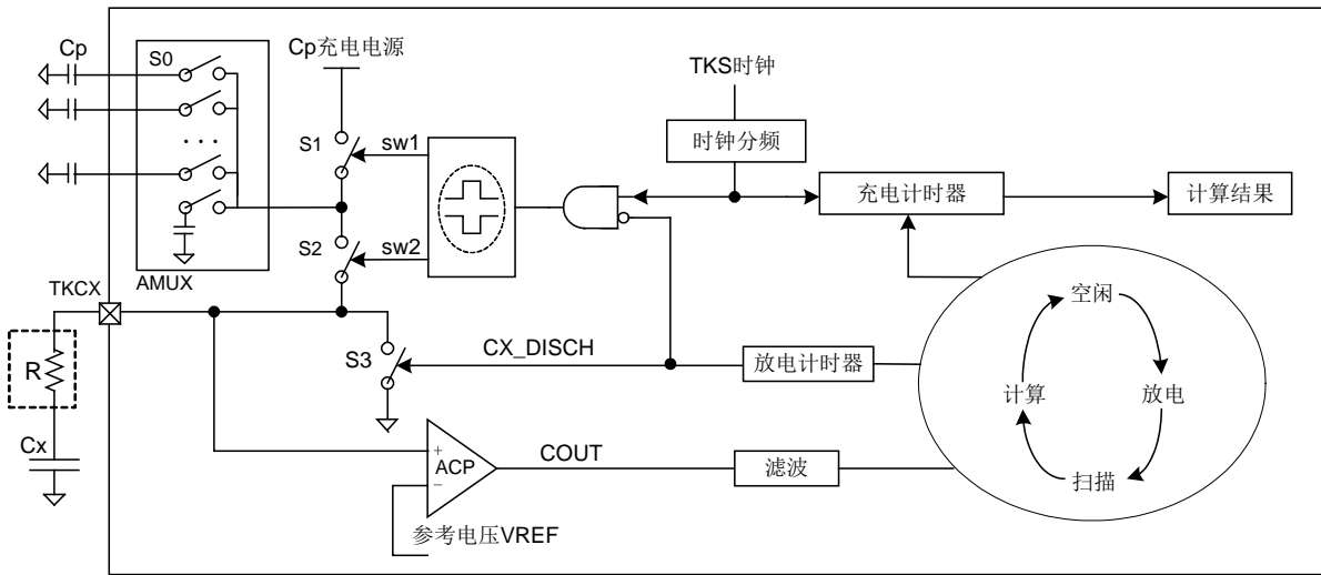
图 5-71 触摸按键充放电结构示意图
