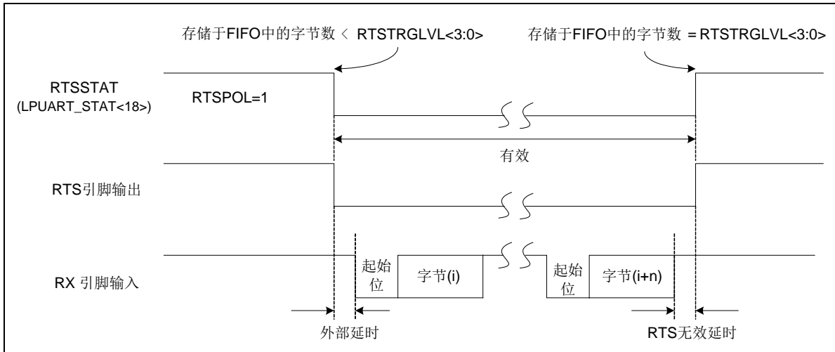
图 5-32 LPUART RTS 自动流控数据接收时序图
