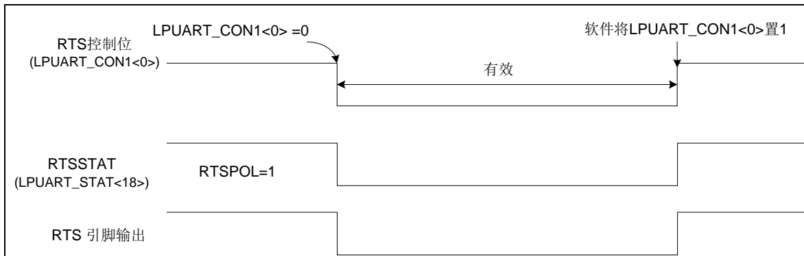
图 5-33 LPUART RTS 软件控制数据接收时序图
