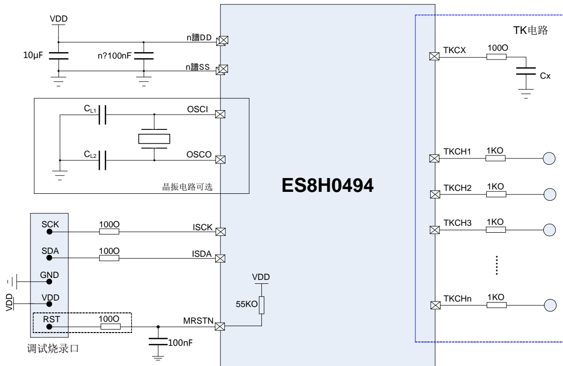
图 1-5 ES8H0494 最小应用系统电路框图
