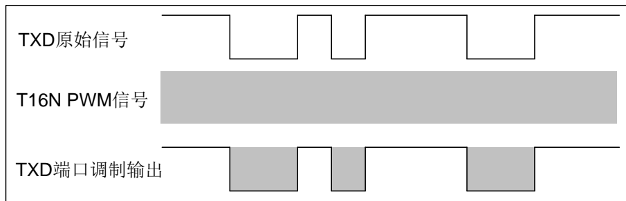
图 5-23 低电平调制输出波形图
