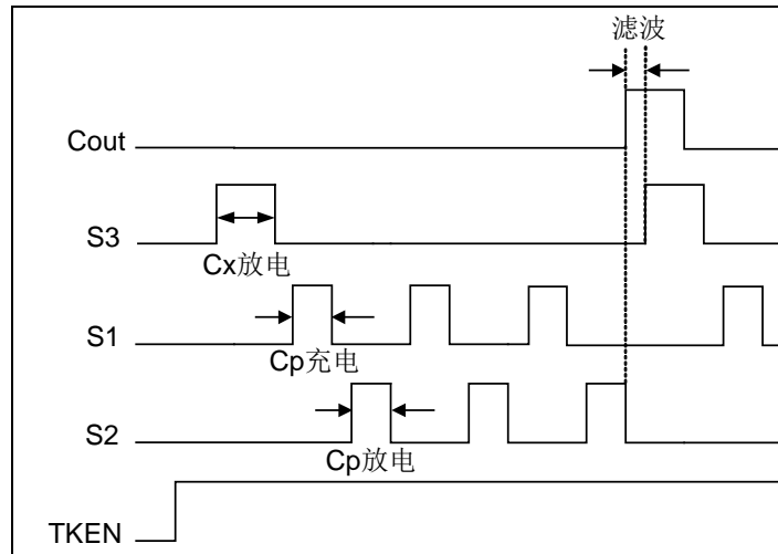
图 5-72 无触摸状态时序图
