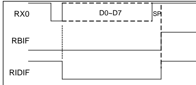
图 5-20 UART 接收中断标志示意图
