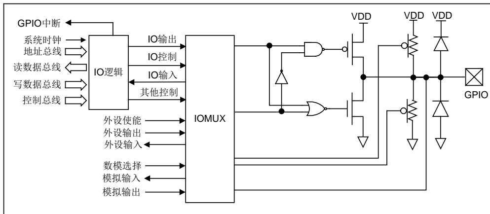
图 4-1 IO 端口电流结构图
