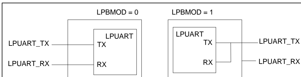
图 5-26 回环模式
