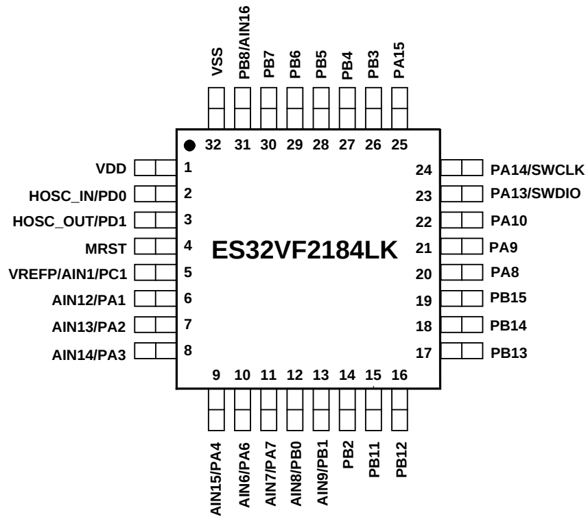
图 3-4 ES32VF2184LK LQFP32 顶视图
