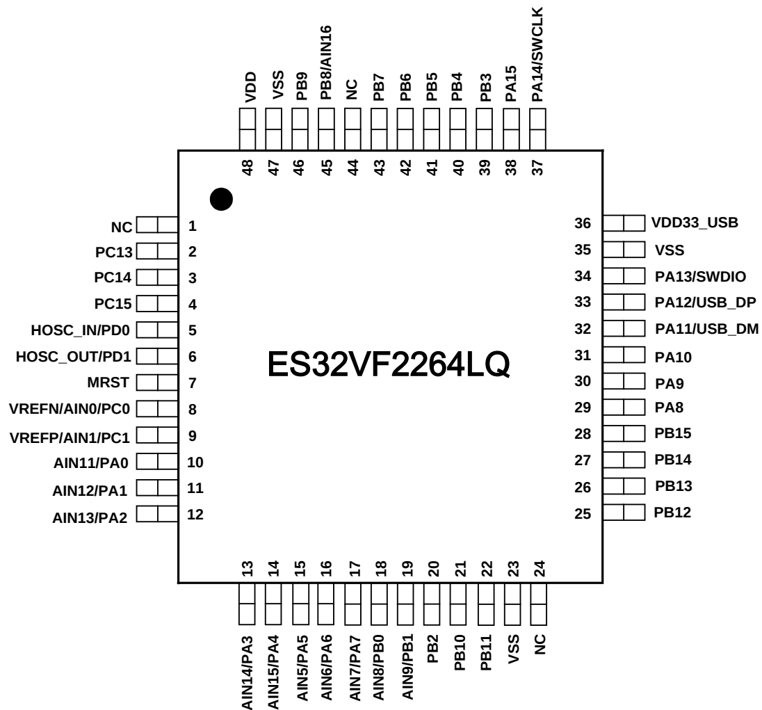
图 3-3 ES32VF2264LQ LQFP48 顶视图
