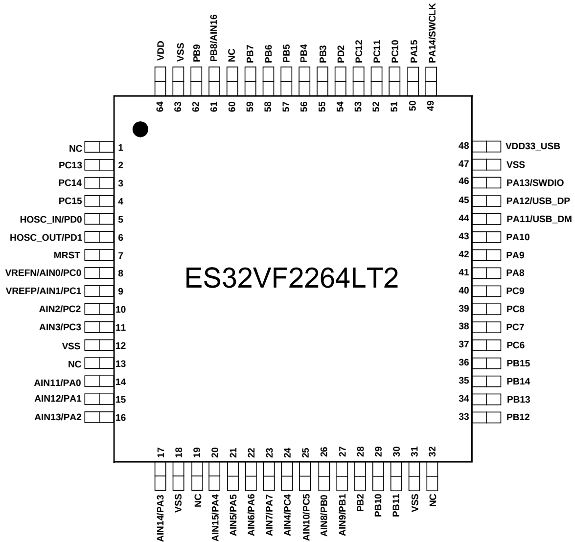
图 3-2 ES32VF2264LT2 LQFP64 顶视图
