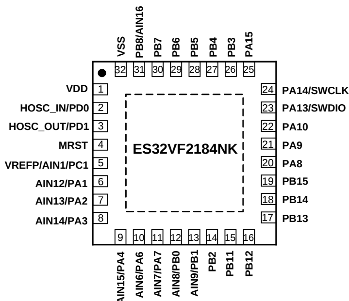
图 3-5 ES32VF2184NK QFN32 顶视图
