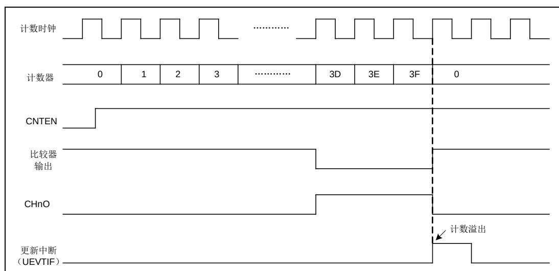
图 17-18 单脉冲模式
