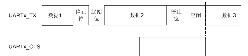
图 22-13 自动 CTSn 控制
