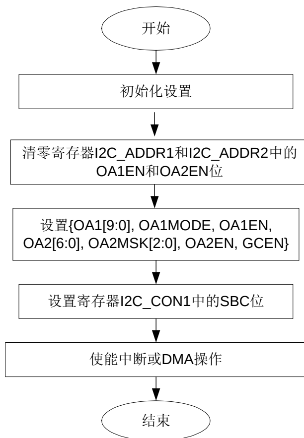
图 20-9 从机初始化流程图
