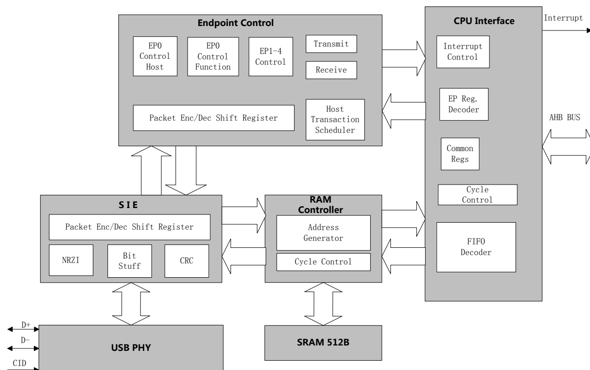
图 23-1 USB 结构图
