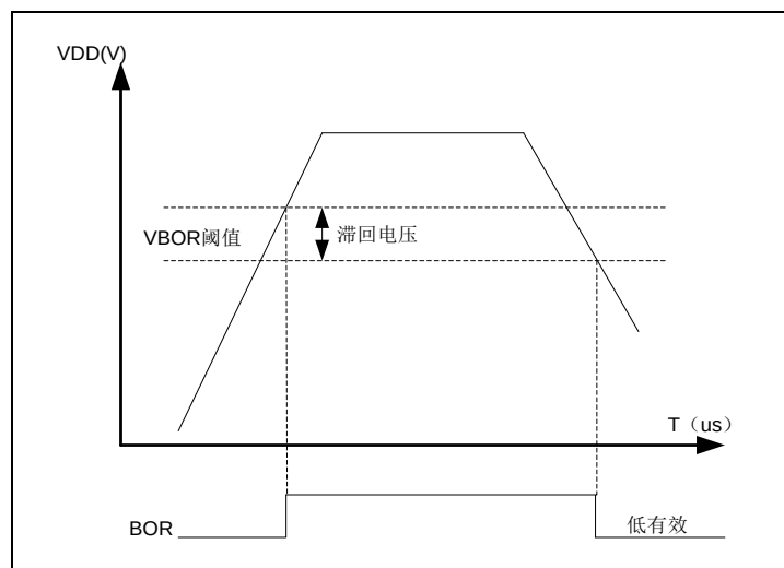
图 7-3 BOR 示意图
