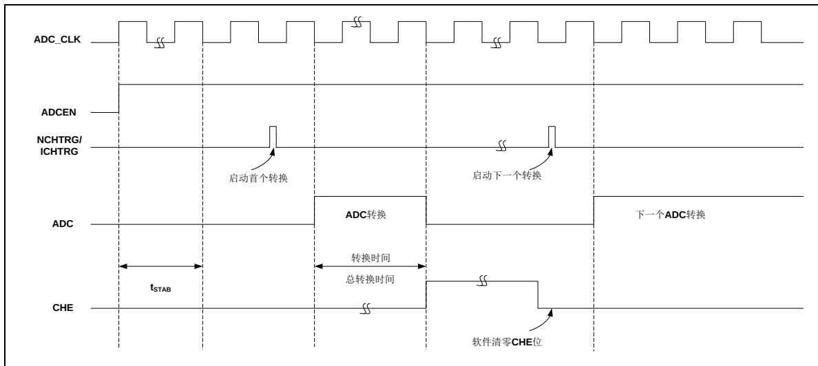
图 24-2 ADC 转换时序图
