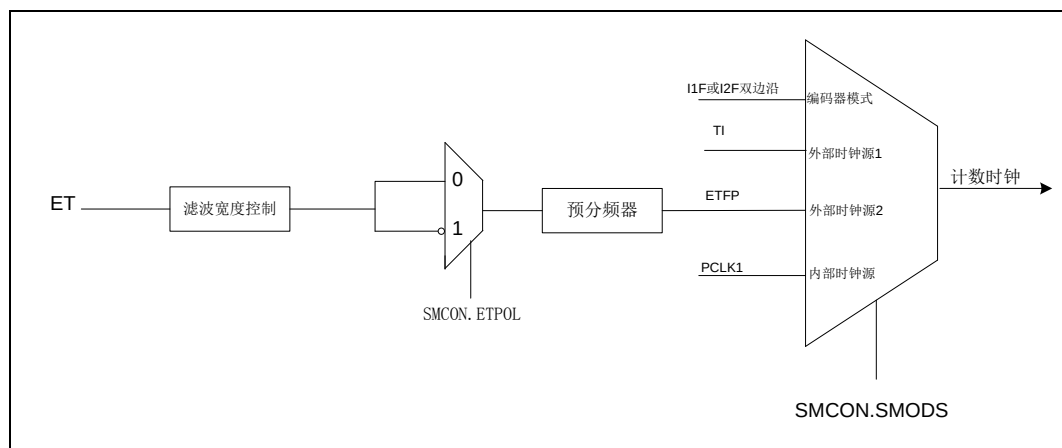
图 18-5 外部触发输入模块
