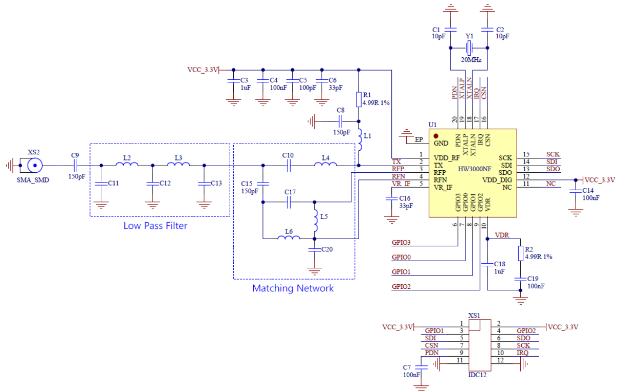
图 13-1 HW3000 典型应用原理图
