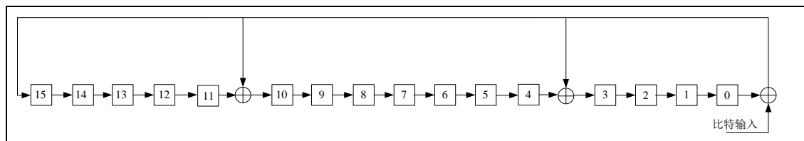
图 12-2 CRC 硬件实现示意图
