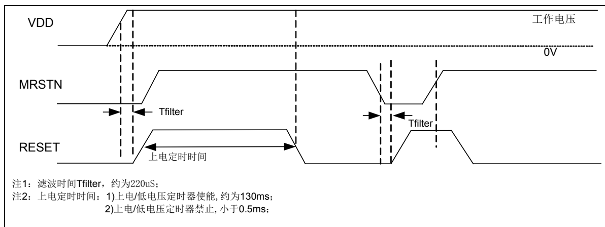
图 5-6 外部 MRSTN 管脚复位
