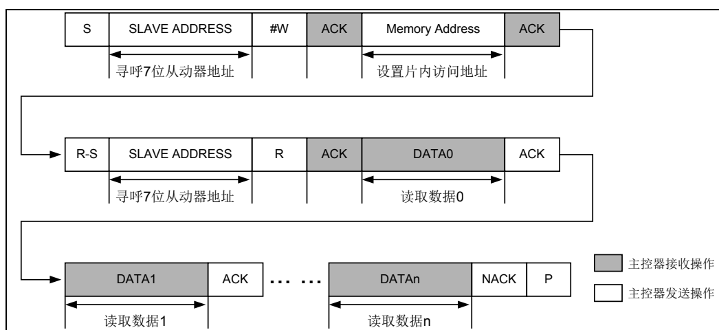
图 6-49 主控器读取从动器数据示意图
