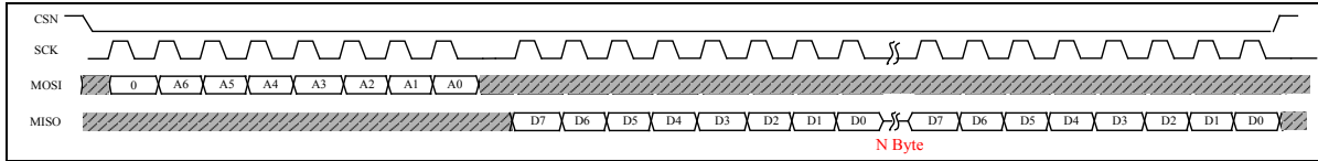
图 14-16 SPI 读 FIFO 时序
