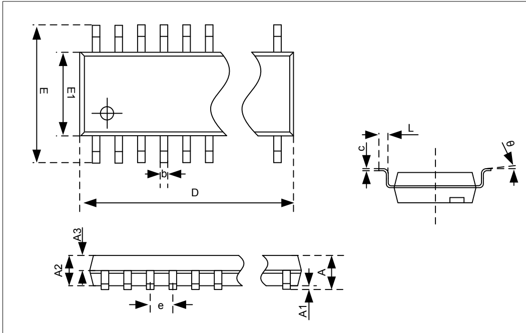
图 18-1 SSOP20 封装图
