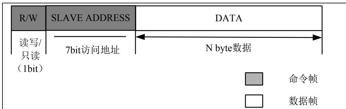
图 14-12 SPI 帧格式
