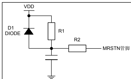
图 5-7 MRSTN 复位参考电路图 1
