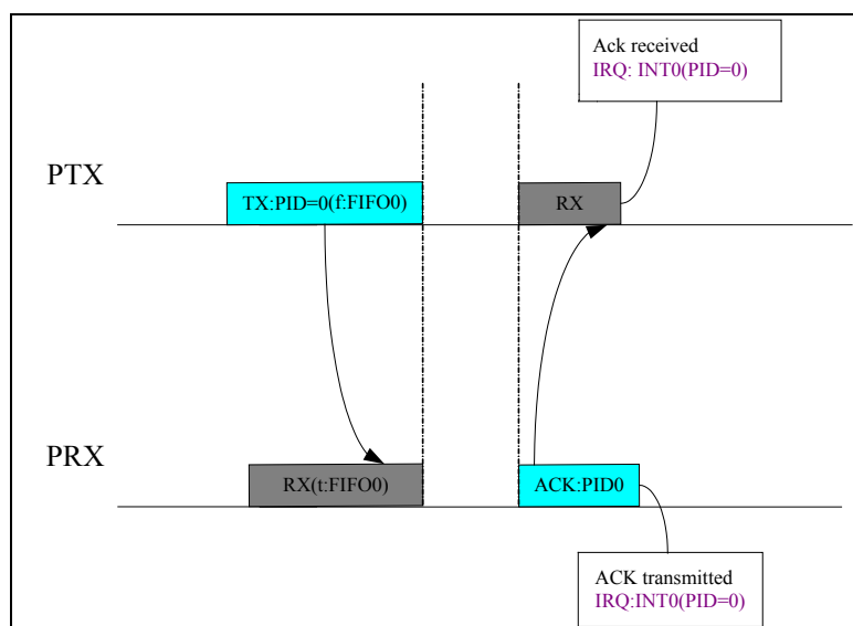
图 14-3 ACK 使能不带 ACK PAYLOAD 中断示意图
