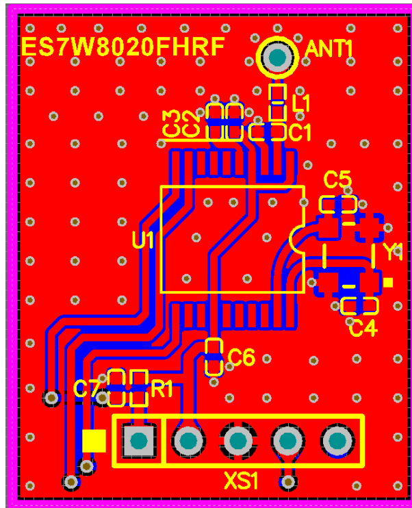
图 19-2 应用参考设计 PCB 图
