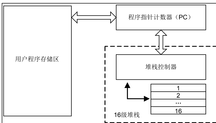
图 3-3 堆栈示意图
