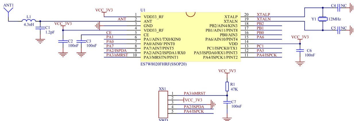
图 19-1 应用参考设计 SCH 图
