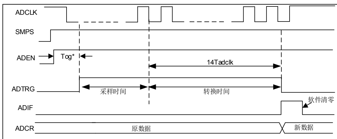
图 6-55 ADC 时序特征示意图 (SMPS=1)
