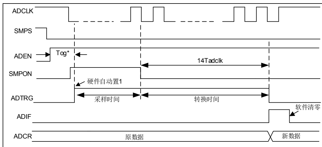
图 6-54 ADC 时序特征示意图 (SMPS=0)
