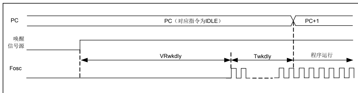
图 5-11 系统唤醒 IDLE 的时序图
