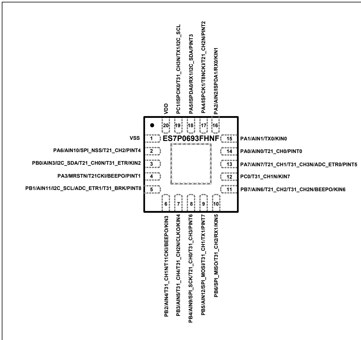
图 1-3 ES7P0693FHNQ 顶视图
