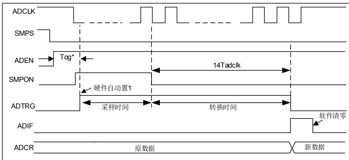
图 6-62 ADC 时序特征示意图 (SMPS=0)
