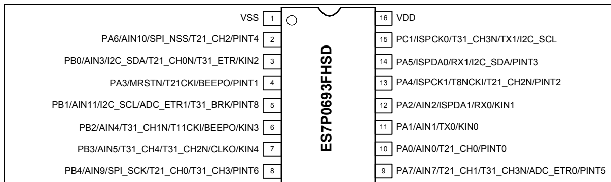
图 1-4 ES7P0693FHSD 顶视图
