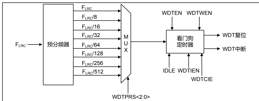
图 5-5 看门狗定时器内部结构图
