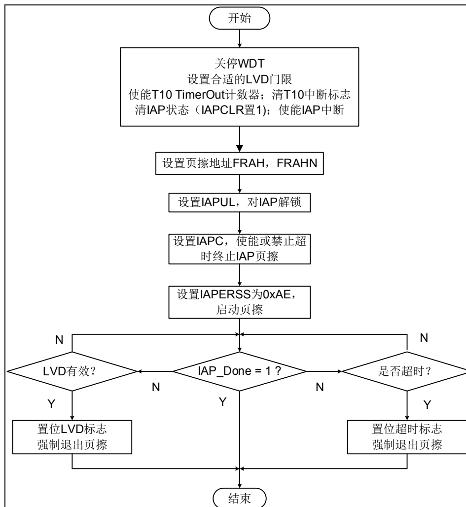
图 3-3 页擦流程图
