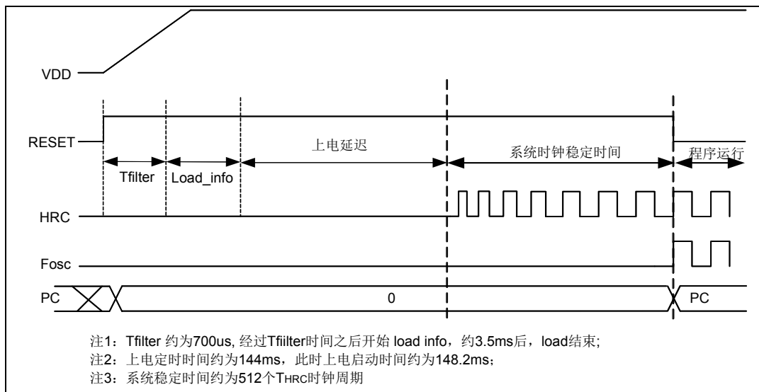
图 5-4 系统上电时序图 2 (MRSTN/PC1 配置为 GPIO)
