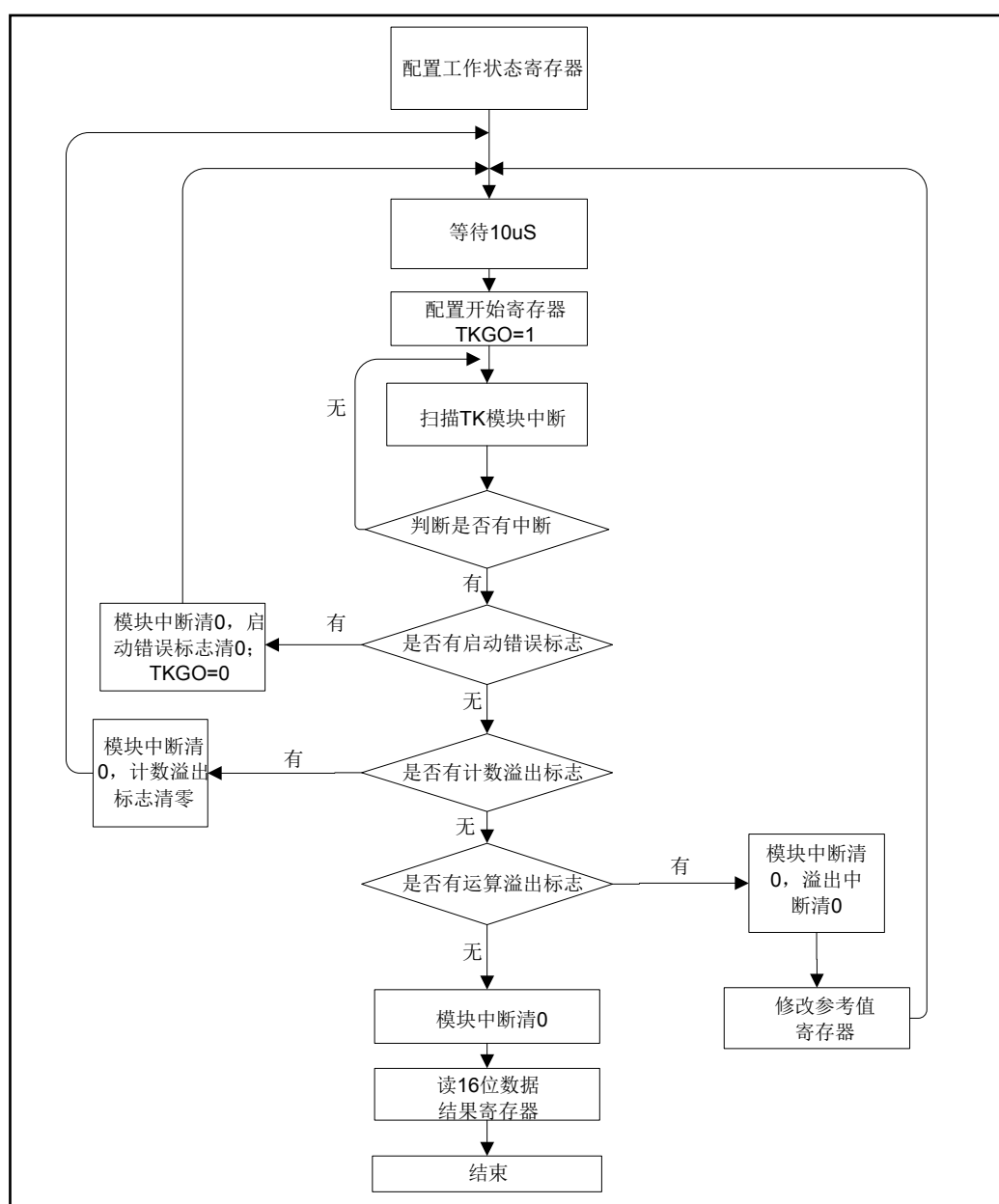
图 6-22 触摸按键操作流程
