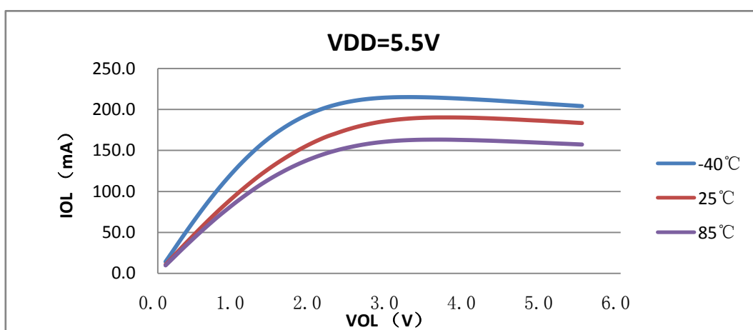
H: V_{OL} vs I_{OL} @VDD=5.5V 大电流端口强驱动模式
