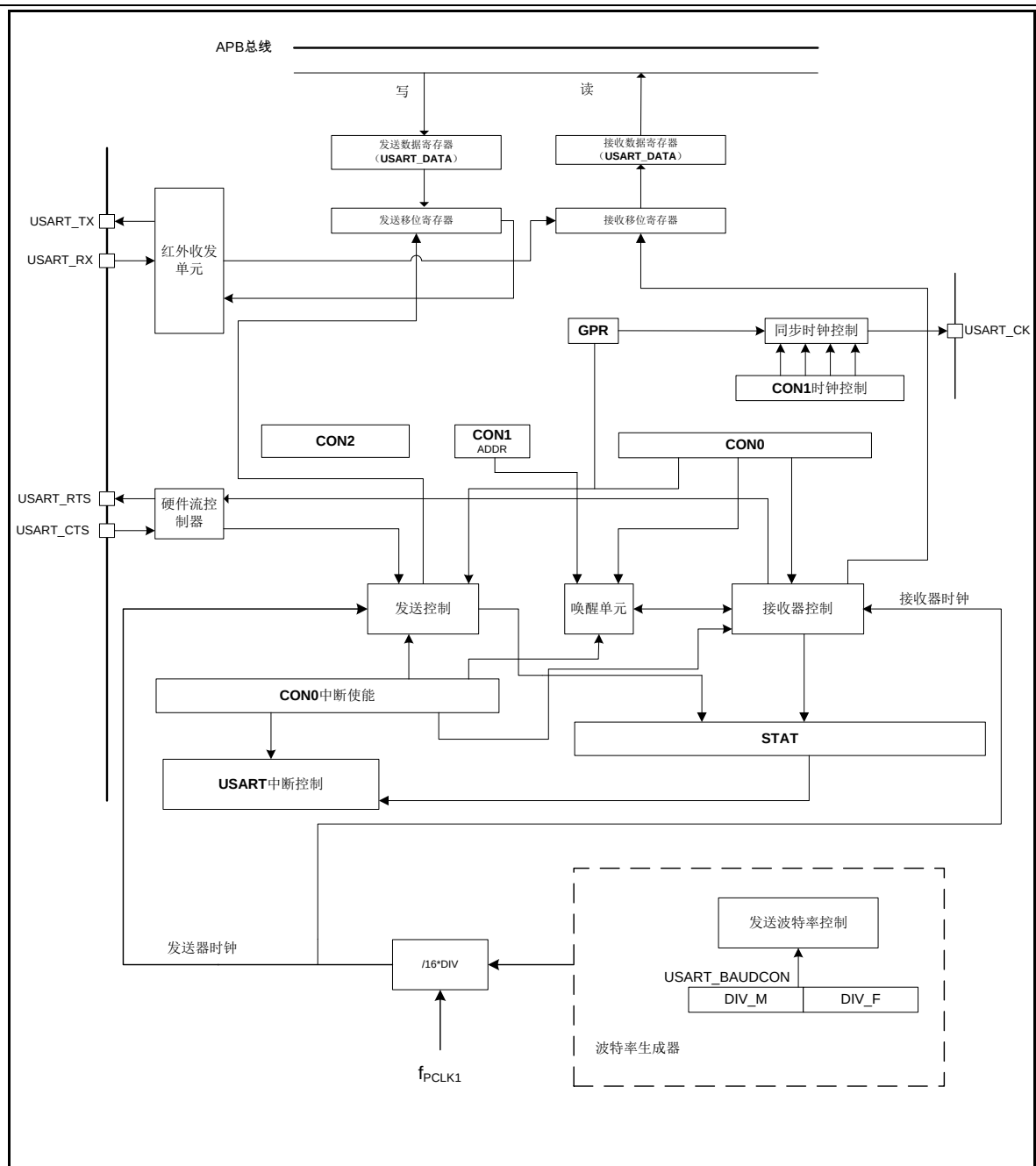
图 27-1 USART 电路结构框图
