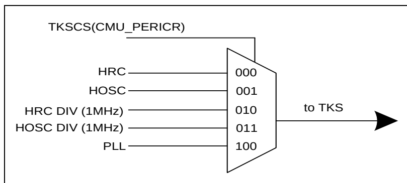
图 3-5 TKS 时钟源
