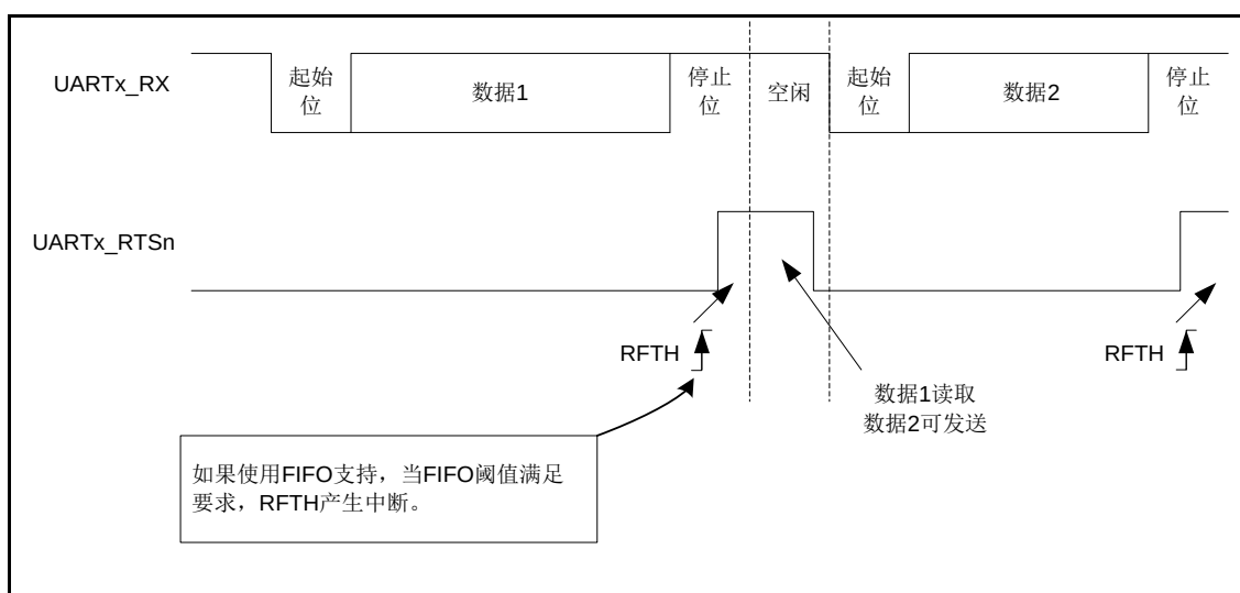
图 26-12 自动 RTSn 控制
