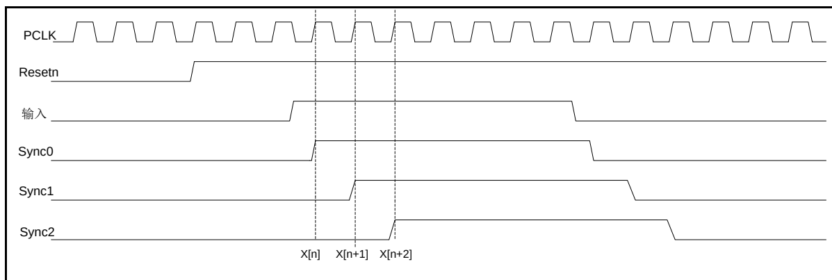
图 26-4 防抖动波形
