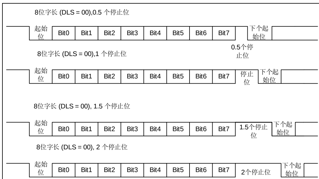
图 26-3 配置停止位
