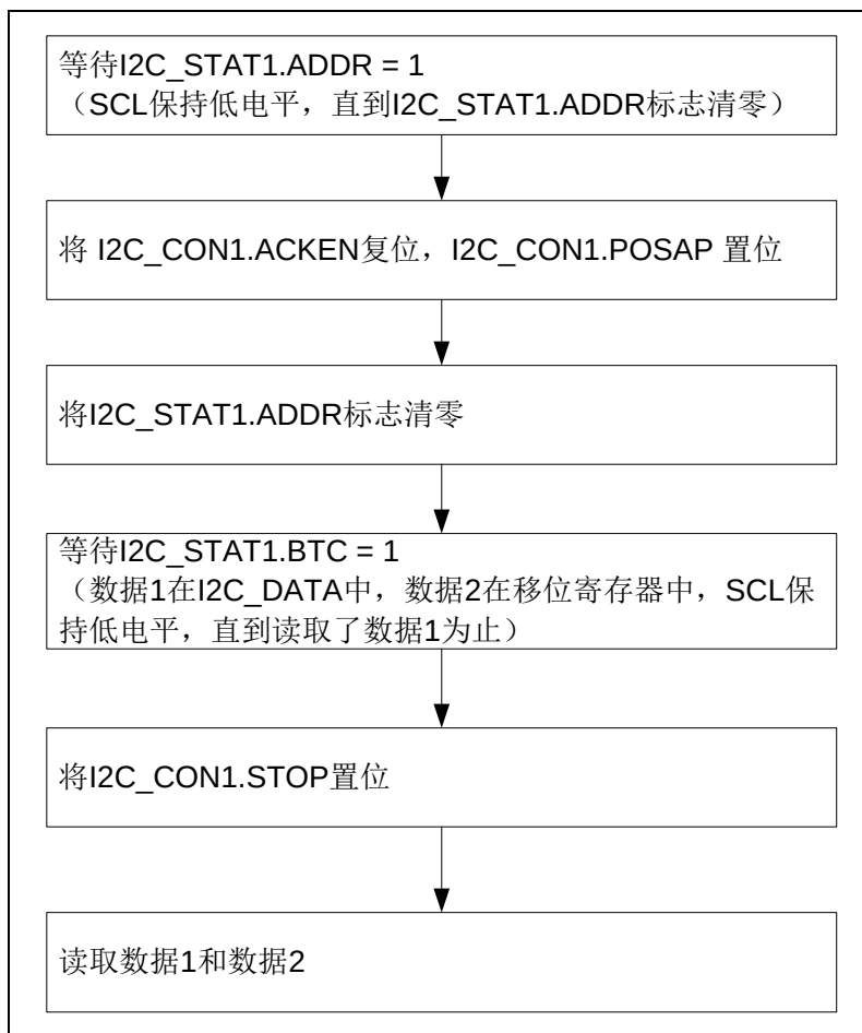
图 24-6 I2C 主模式 2 字节接收
