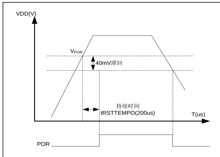
图 7-2 POR 示意图
