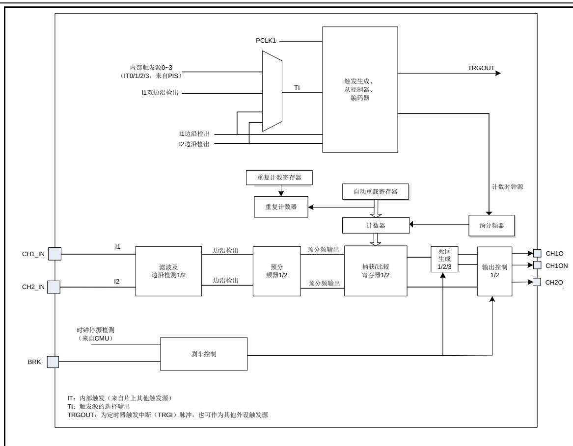
图 20-1 通用定时器 GP16C2T 结构框图
