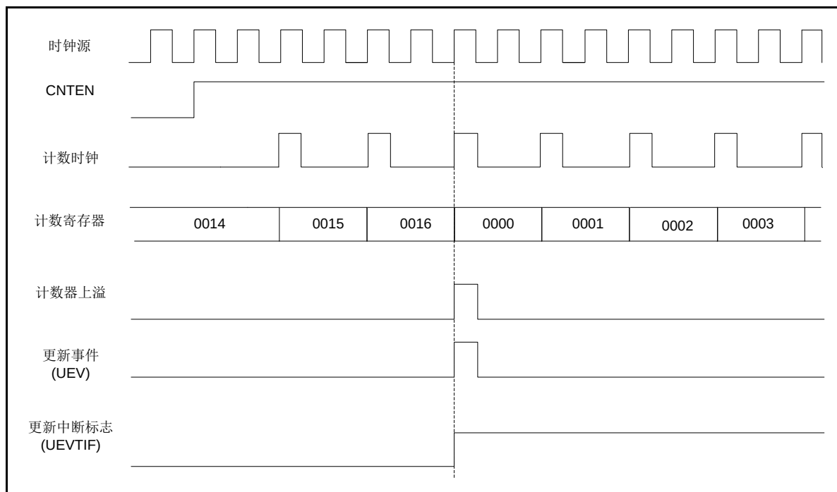
图 20-6 计数器递增计数时序图
