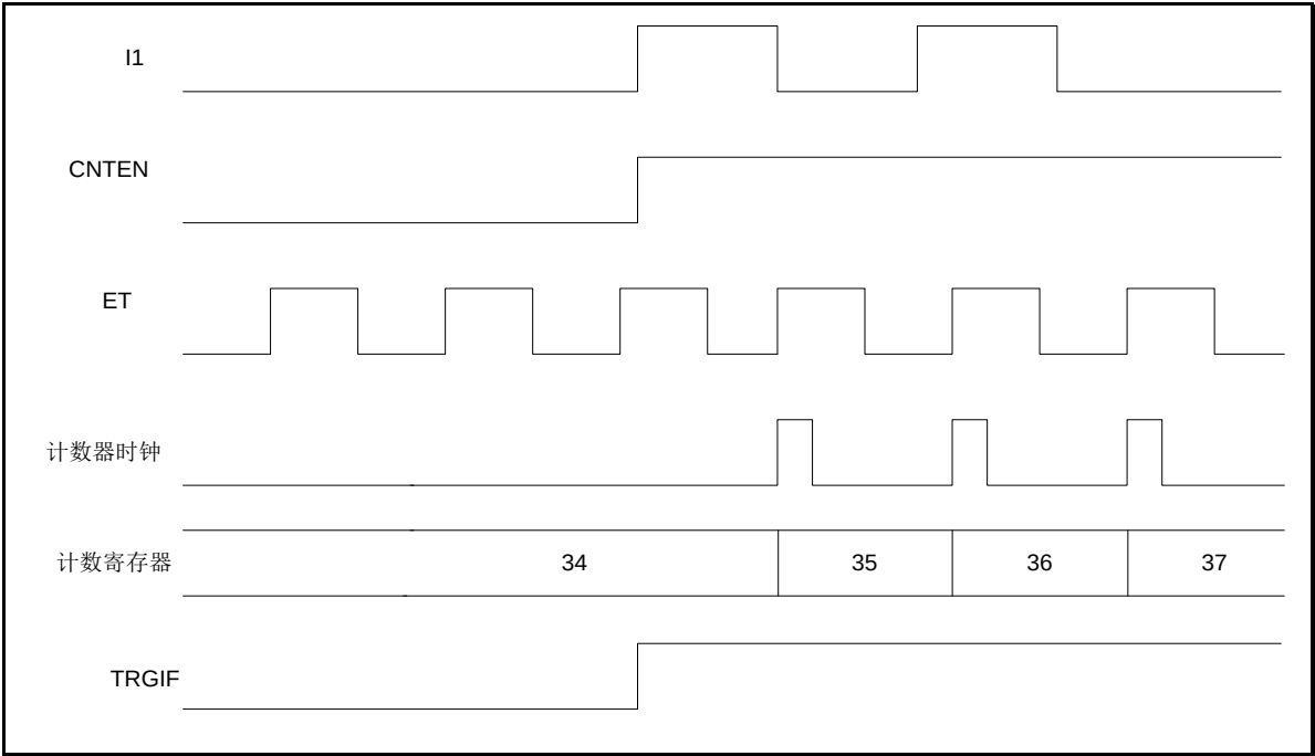
图 19-24 外部时钟源 2+触发模式下的控制电路
