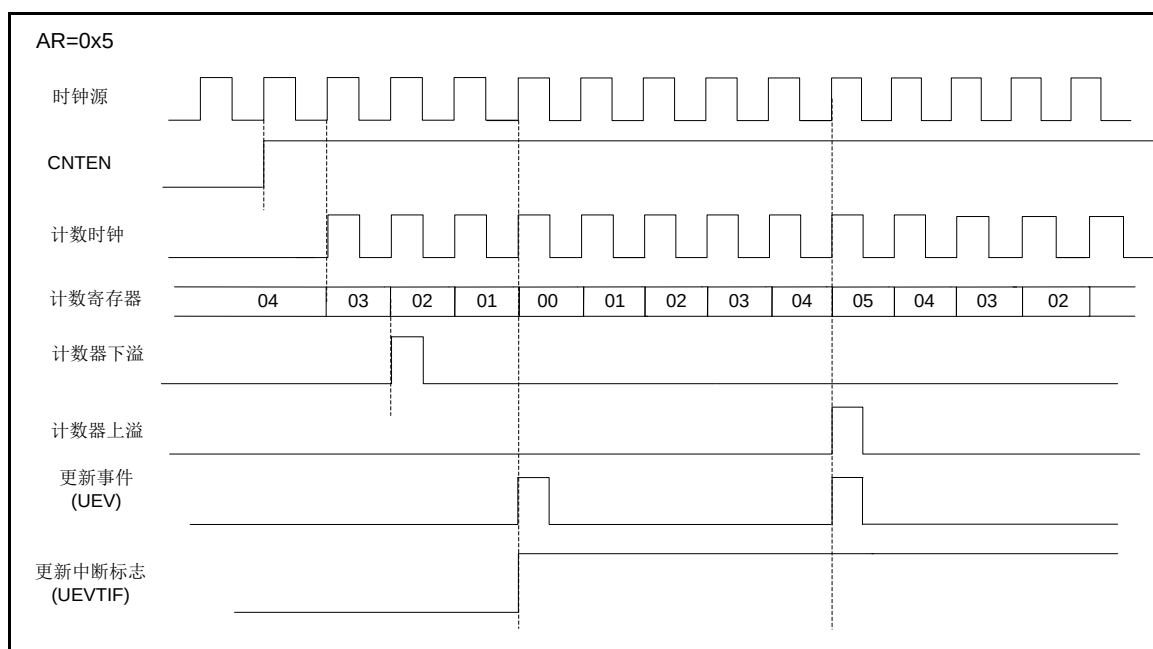
图 19-11 增减计数器时序图
