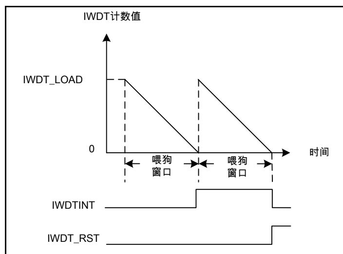
图 12-1 独立看门狗时序图
