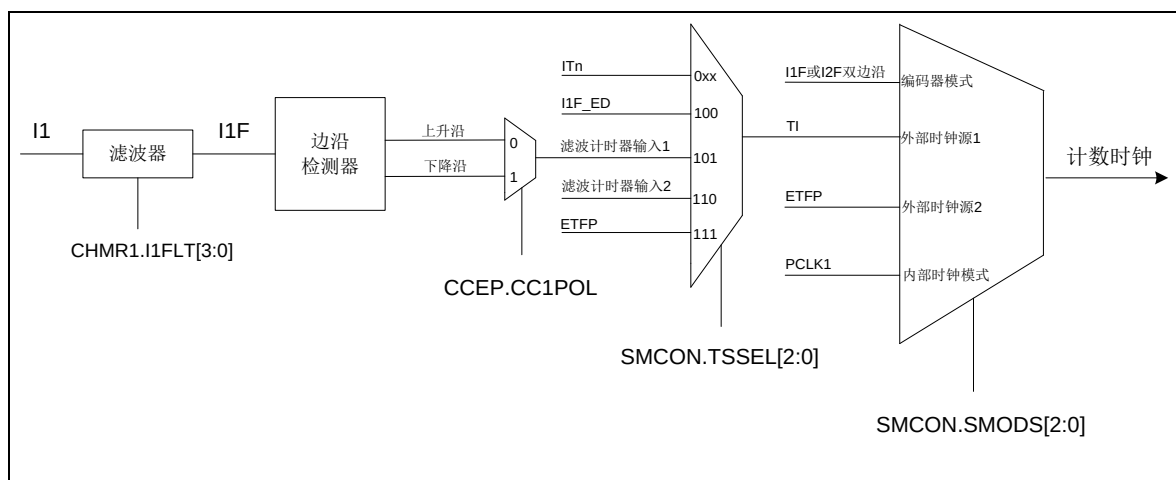
图 19-4 I1 外部时钟连接
