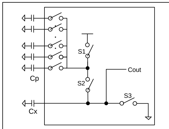
图 15-2 充放电开关示意图
