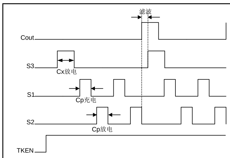
图 15-4 方案 A 有触摸状态内部时序图
