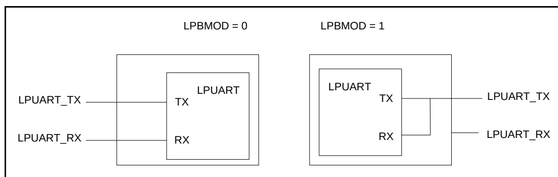
图 28-14 回环模式
