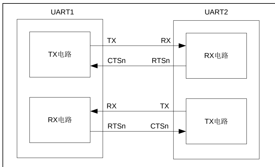
图 26-11 自动流控制框图
