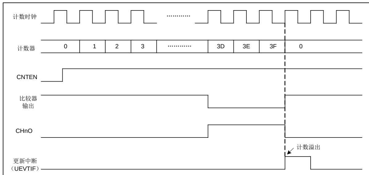
图 20-15 单脉冲模式
