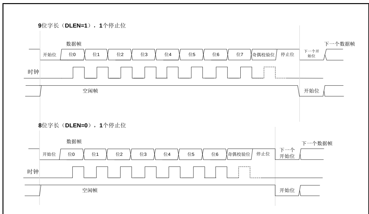
图 27-2 USART 帧格式
