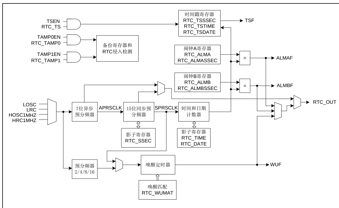
图 23-1 电路结构框图
