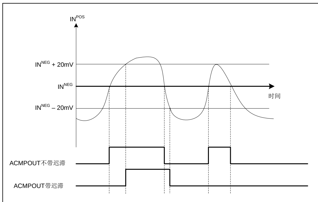
图 30-2 迟滞原理图
