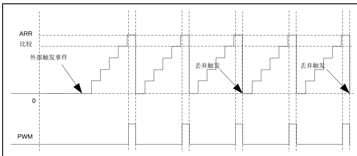
图 22-4 连续计数
