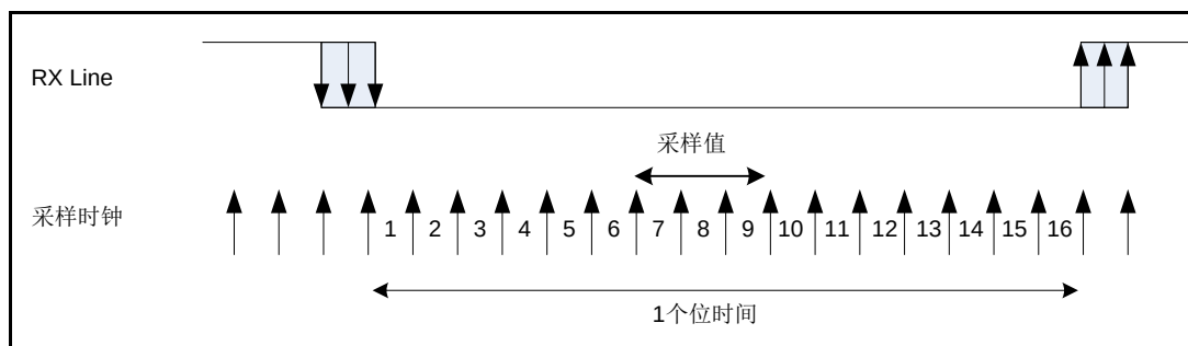
图 26-7 数值采样
