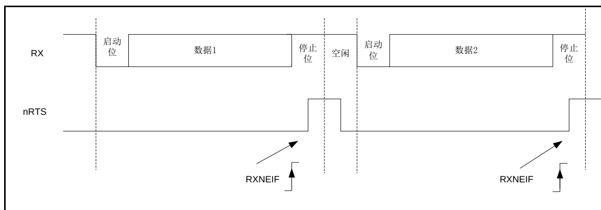
图 27-18 RTS 流控制
