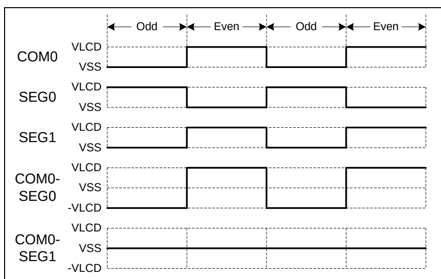
图 16-4 静态占空比波形图
