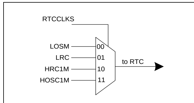
图 3-7 RTC 计数时钟
