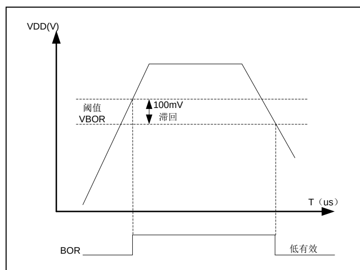
图 7-3 BOR 示意图
