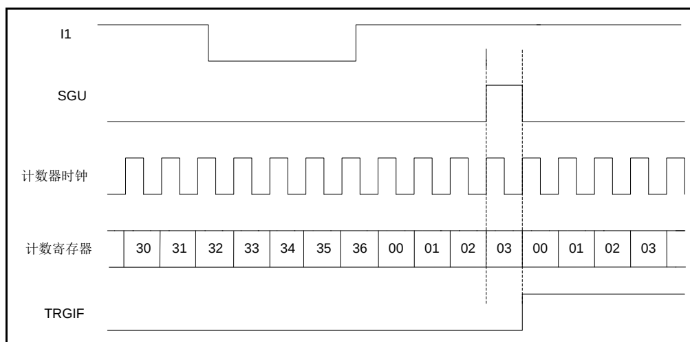
图 19-21 复位模式控制电路
