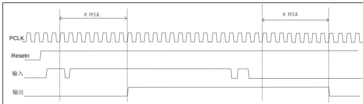
图 26-5 防抖动输出
