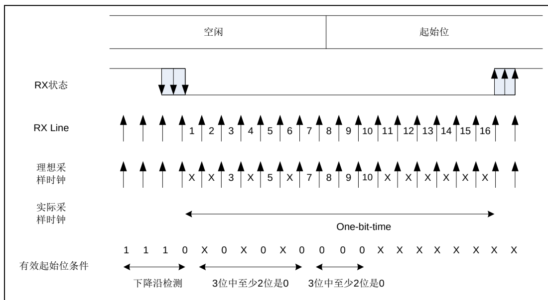
图 26-6 起始位检测
