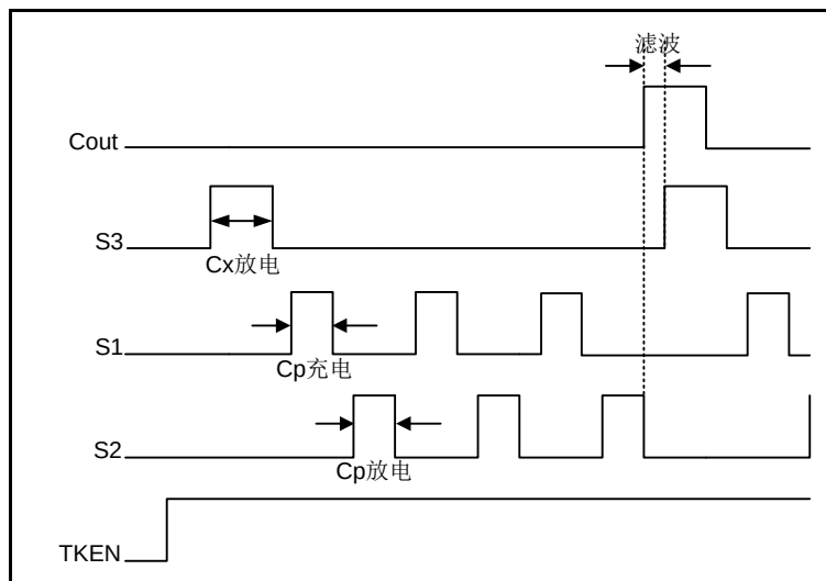
图 15-3 方案 A 无触摸状态内部时序图
