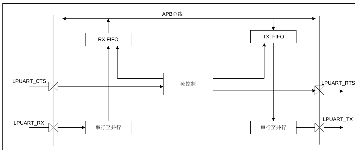
图 28-6 LPUART 自动流控制
