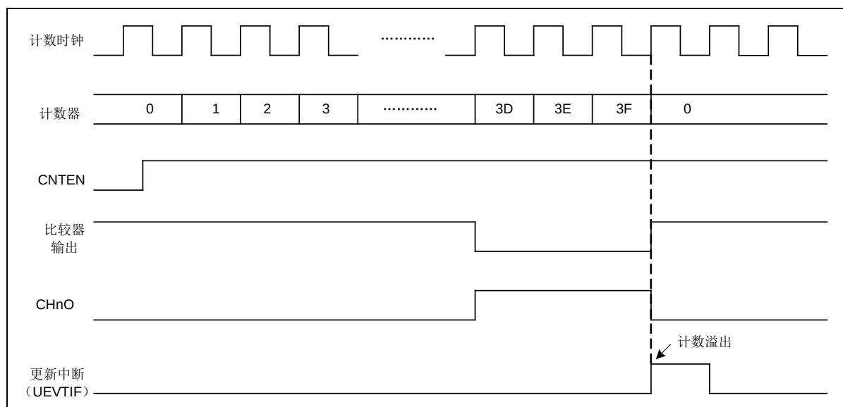
图 19-18 单脉冲模式
