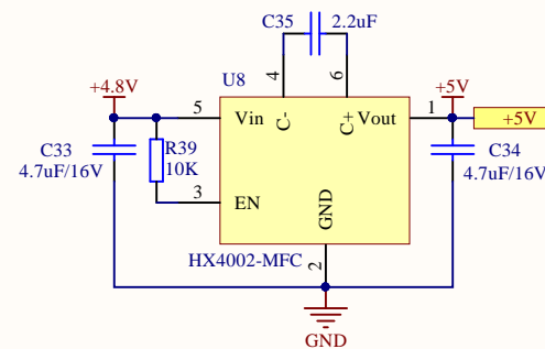
5V电压泵升电路
