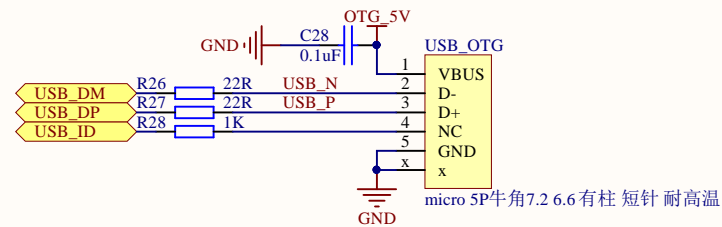
USB-OTG接口
