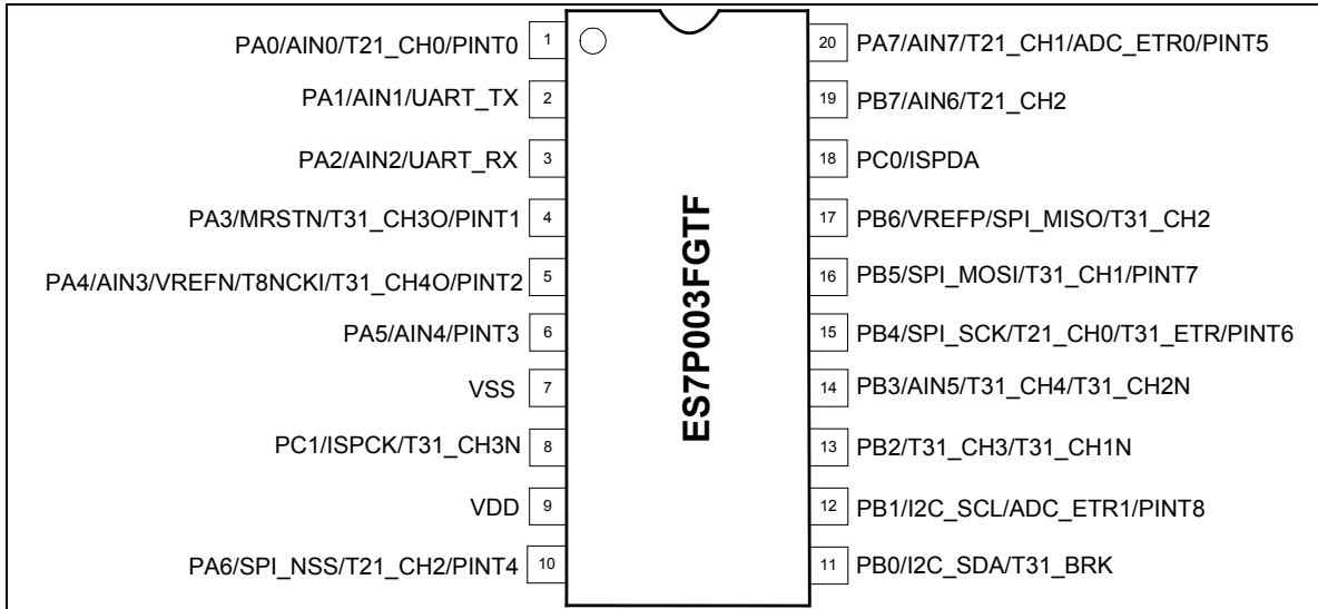
图 1-2 ES7P003FGTF 顶视图
