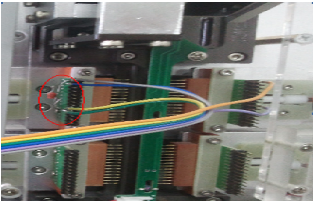
图表 2-4 ISP 烧录连接连接图示二
