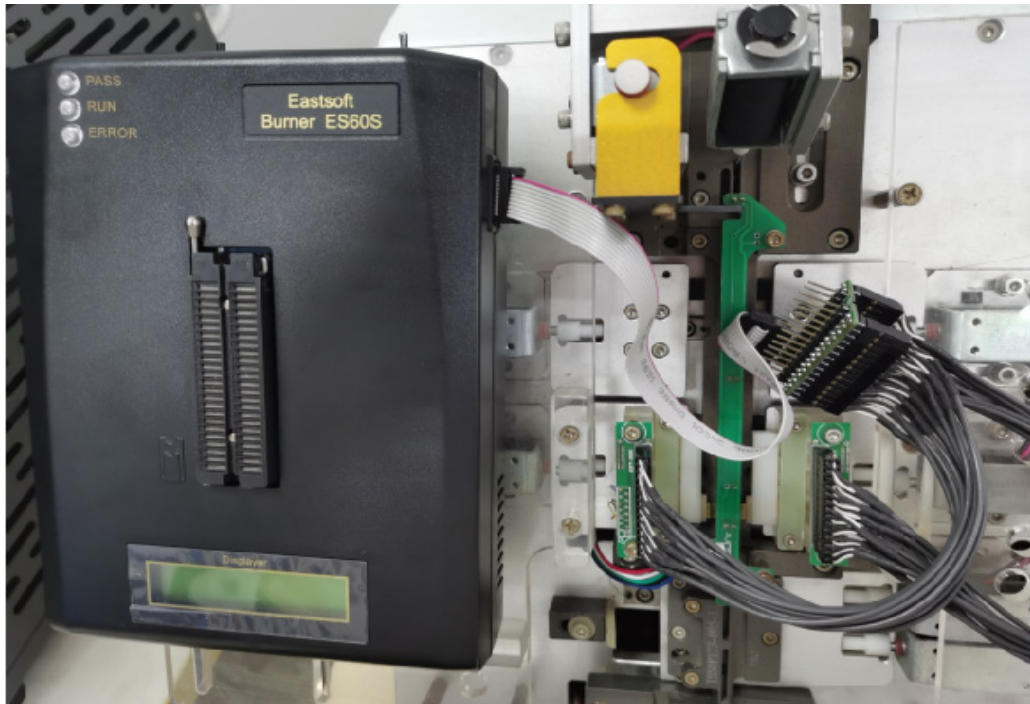
图表 2-3 ISP 烧录连接图示一
