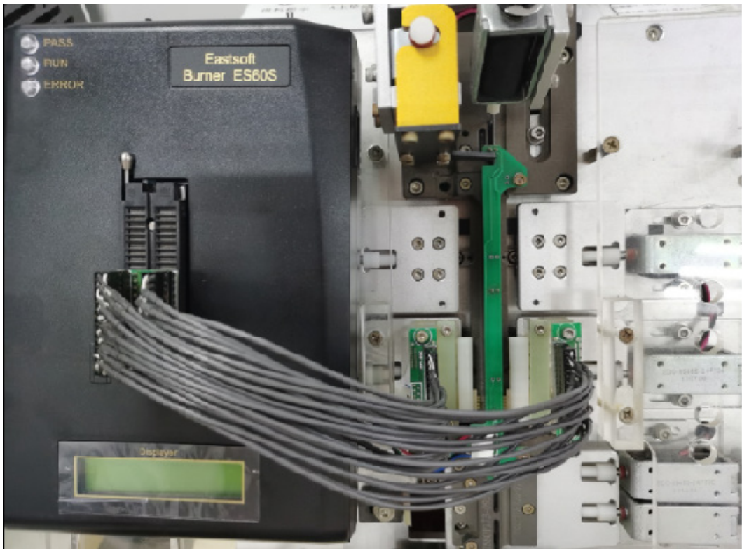
图表 2-2 锁紧座烧录连接图示
