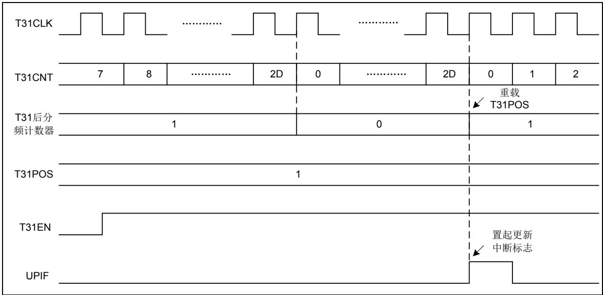
图 6-14 使用后分频的计数时序图 (T31CNTLD=0x2D)
