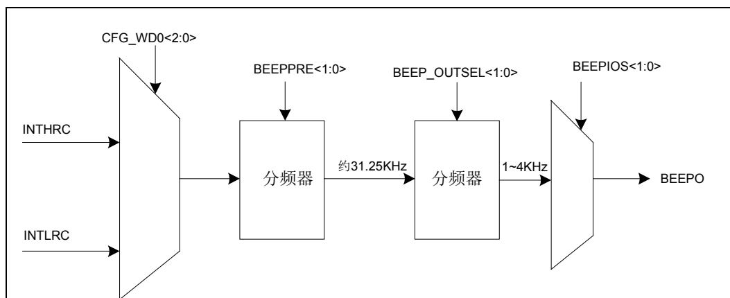
图 5.1 BEEPER 结构图
