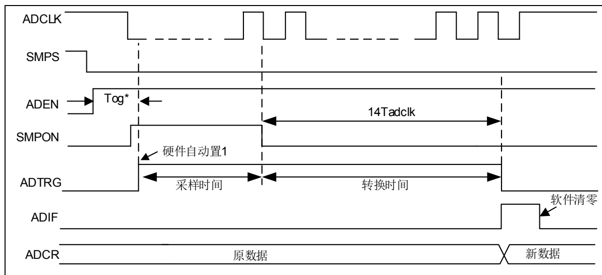
图 6-62 ADC 时序特征示意图 (SMPS=0)
