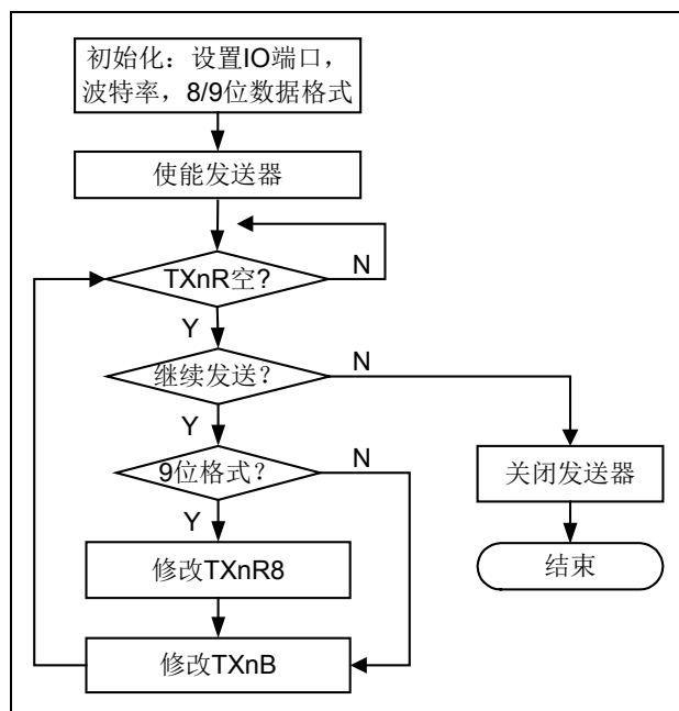
图 6-38 UARTn 发送器操作流程图中
