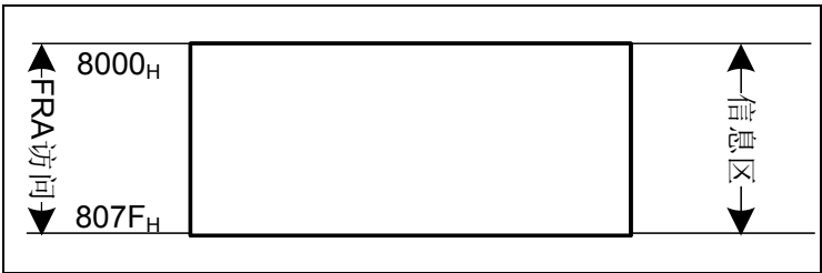
图 3-3 信息区寻址空间映射图
