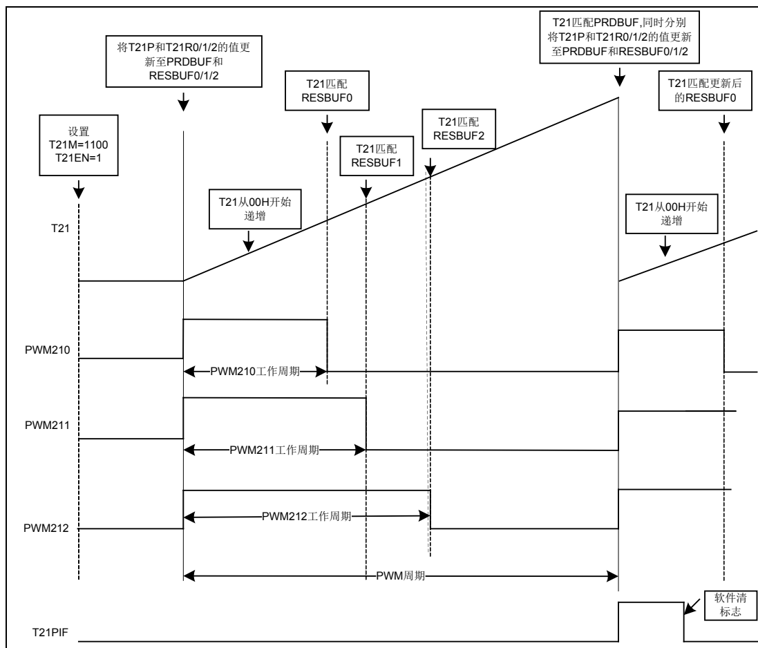
图 6-9 T21 多精度 PWM 模式示意图
