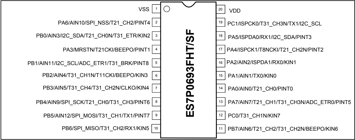
图 1-2 ES7P0693FHT/SF 顶视图
