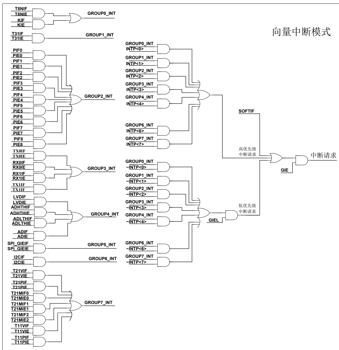
图 7-2 向量中断模式中断控制逻辑
