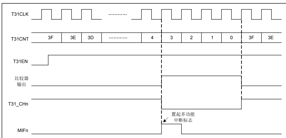
图 6-26 普通 PWM 波形，递减计数 (T31CHnR=3, T31CNTLD=0x3F, CHnP=1)
