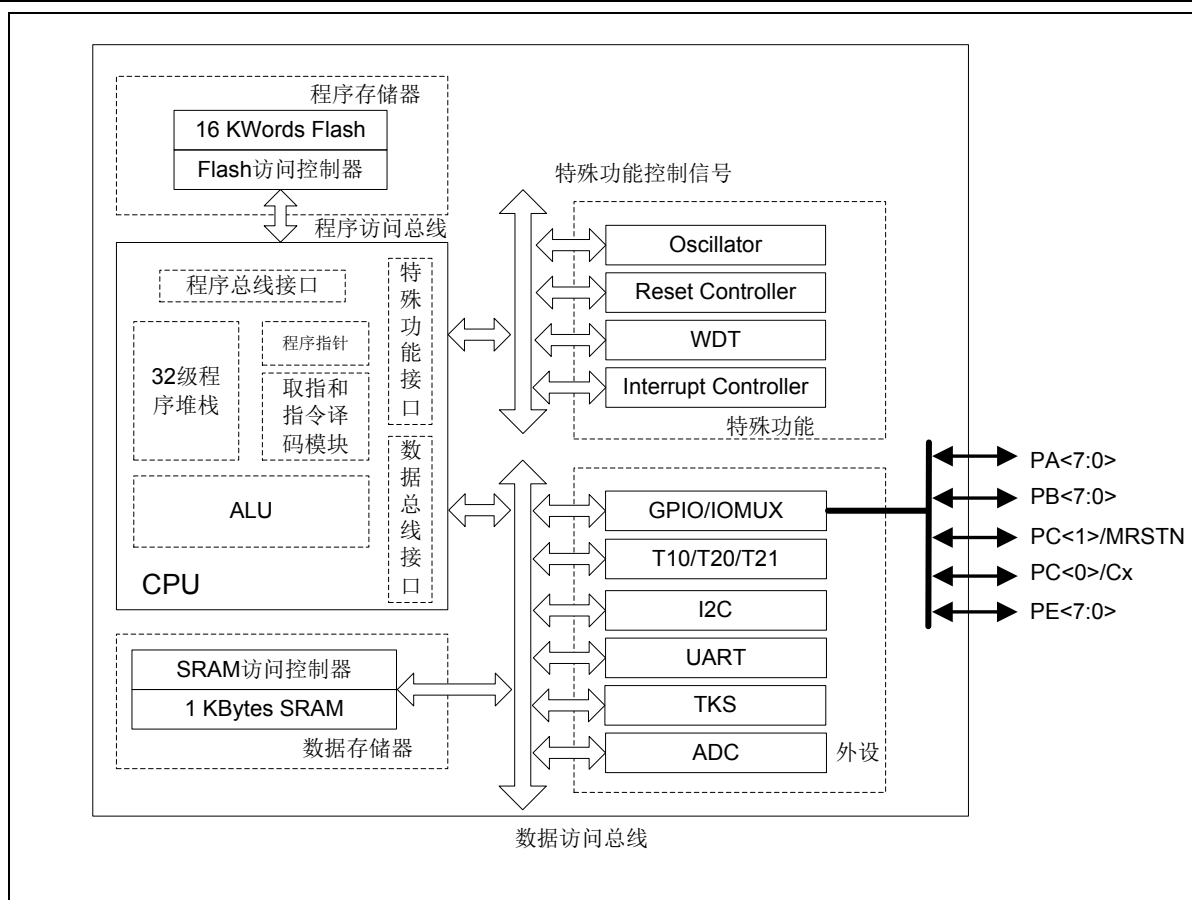
图 1-1 结构框图
