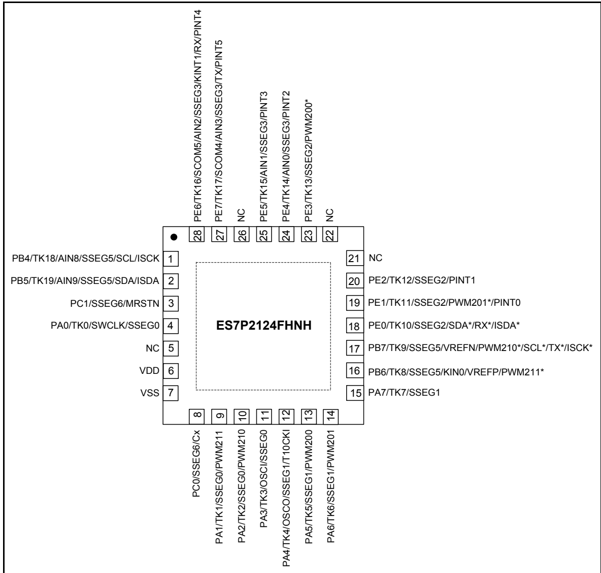
图 1-2 QFN28 封装顶视图
