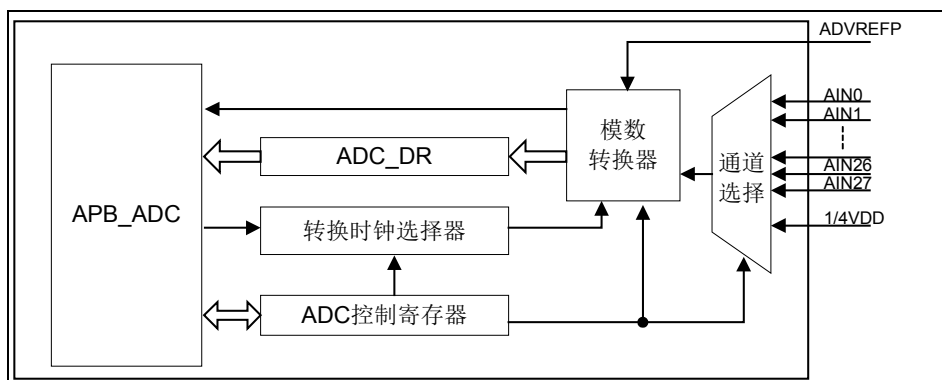
图 5-41 ADC 内部结构图
