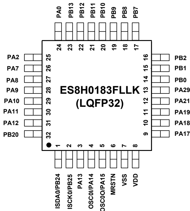
图 1-9 ES8H0183FLLK LQFP32 封装顶视图
