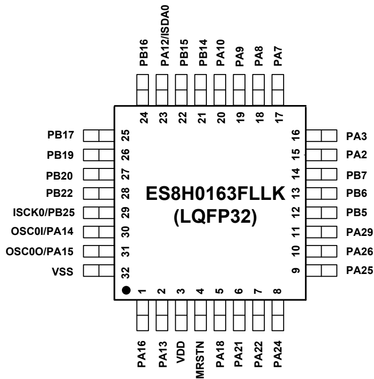
图 1-7 ES8H0163FLLK LQFP32 封装顶视图
