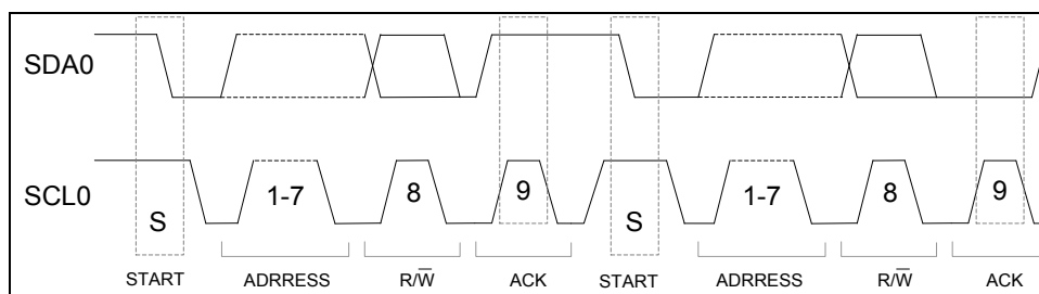
图 5-36 I2C 自动寻呼波形图
