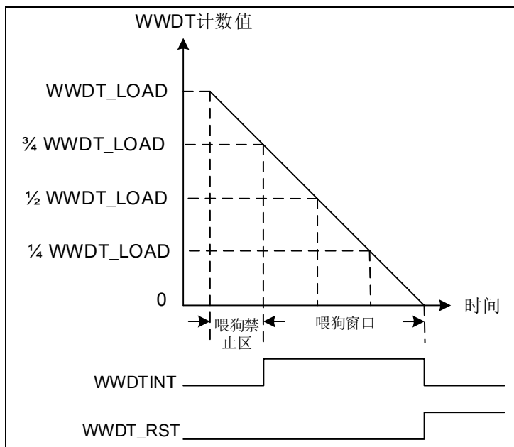
图 5-45 窗口看门狗中断和溢出复位产生时序图 (WWDTWIN 设定为 25%)
