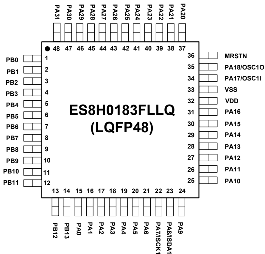
图 1-4 ES8H0183FLLQ LQFP48 封装顶视图
