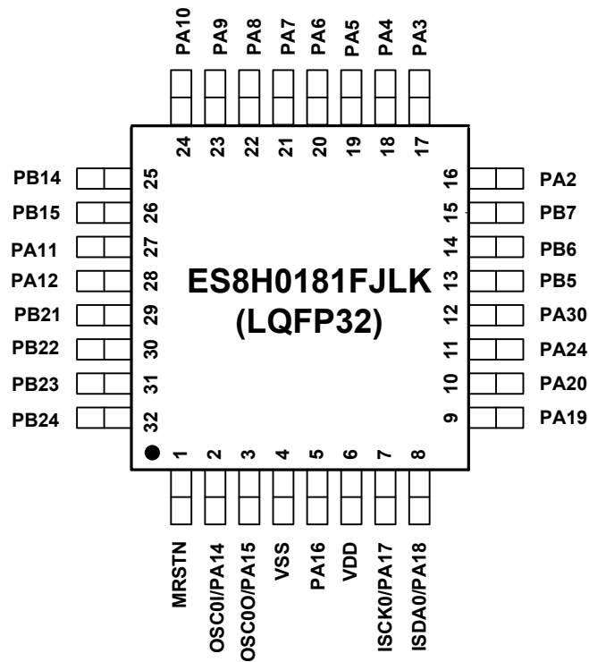
图 1-8 ES8H0181FJLK LQFP32 封装顶视图
