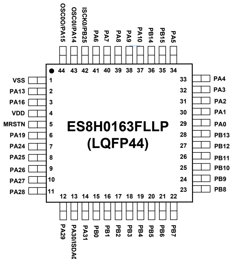
图 1-6 ES8H0163FLLP LQFP44 封装顶视图
