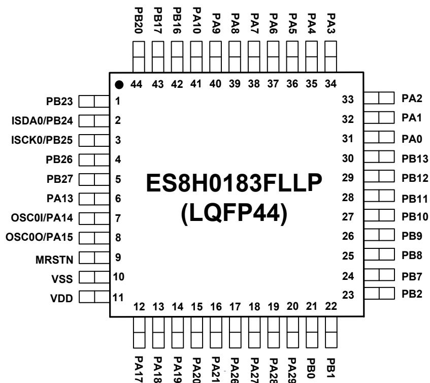
图 1-5 ES8H0183FLLP LQFP44 封装顶视图
