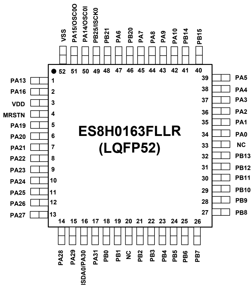
图 1-3 ES8H0163FLLR LQFP52 封装顶视图
