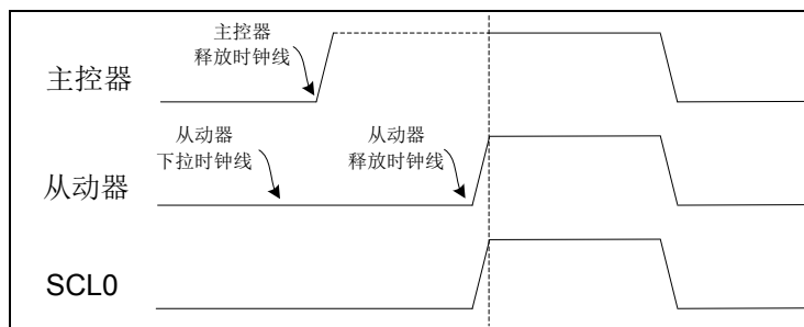
图 5-40 I2C 时钟线下拉等待波形示意图
