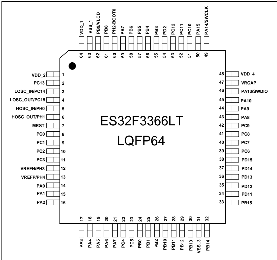
图 3-2 ES32F3366 LQFP64 顶视图
