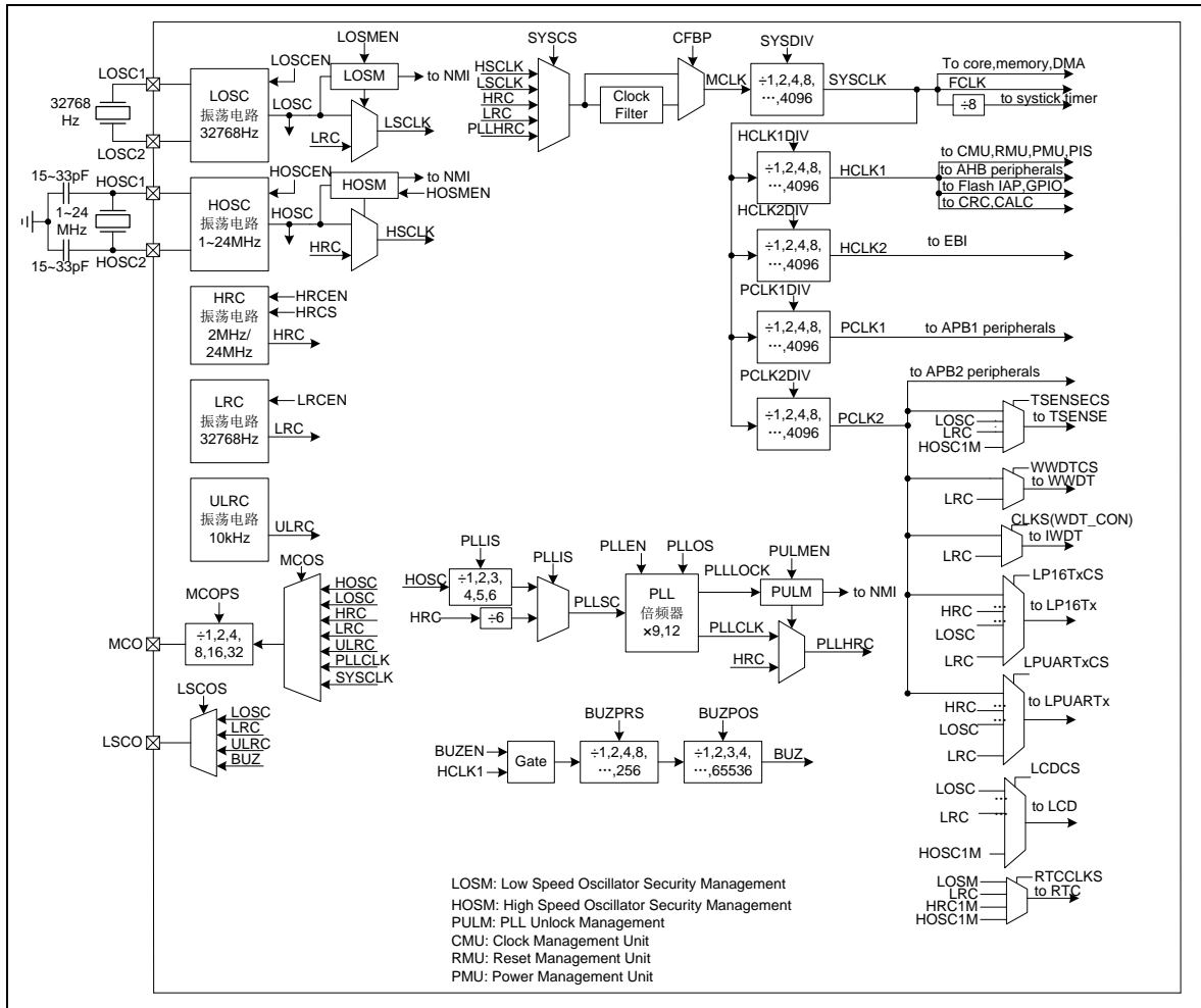
图 2-2 时钟树
