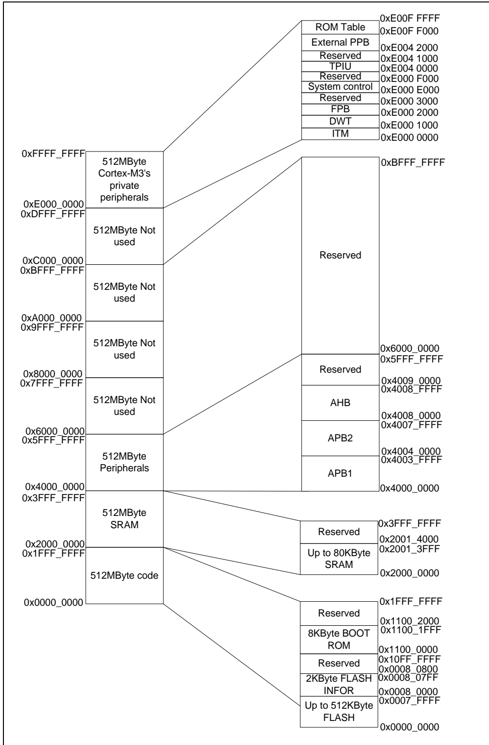
图 4-1 存储器映射
