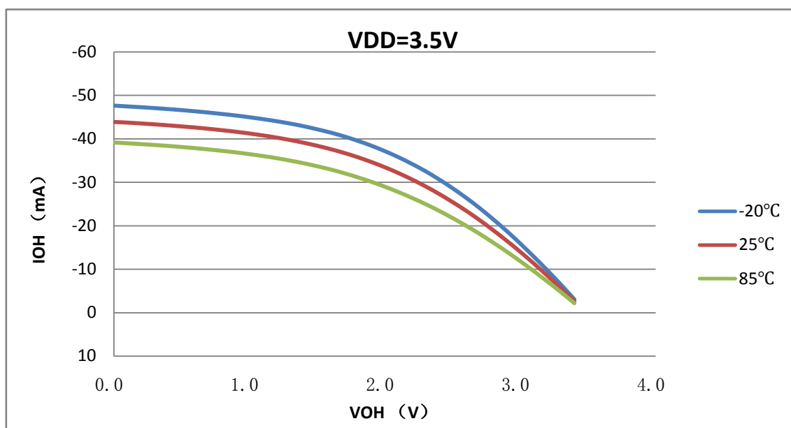
◇ I_{OH} vs V_{OH} @VDD=3.5V (驱动 2)
