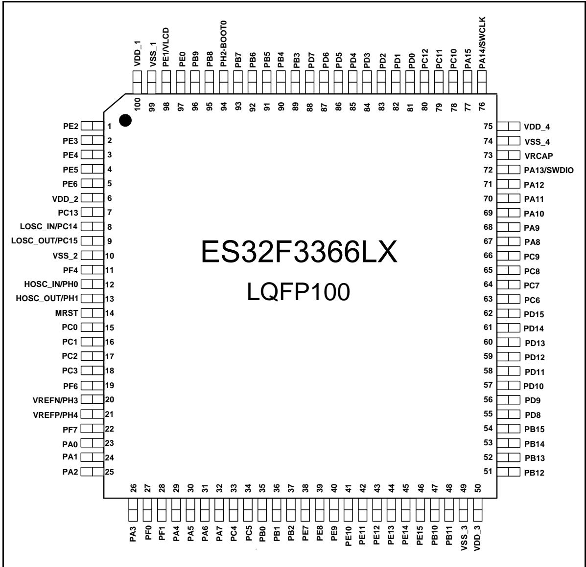
图 3-1 ES32F3366 LQFP100 顶视图
