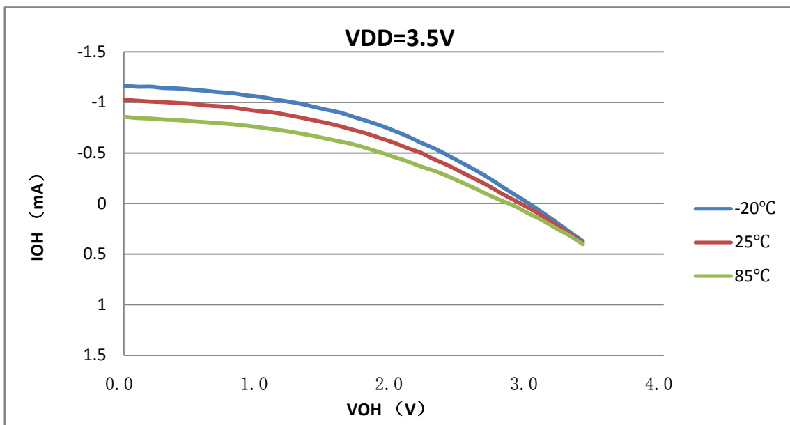
◇ I_{OH} vs V_{OH} @VDD=3.5V (驱动 0)
