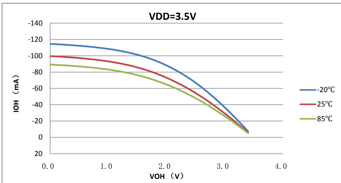
◇ I_{OH} vs V_{OH} @VDD=3.5V (驱动 3)
