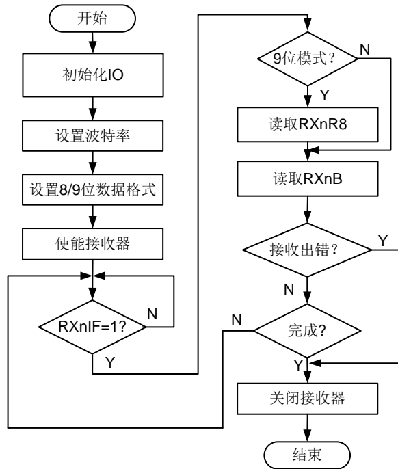
图 6-12 UARTn 接收器操作流程图
