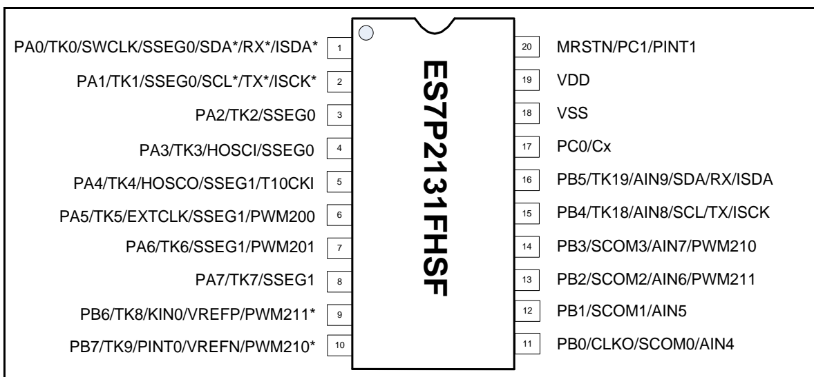
图 1-3 SOP20 封装顶视图
