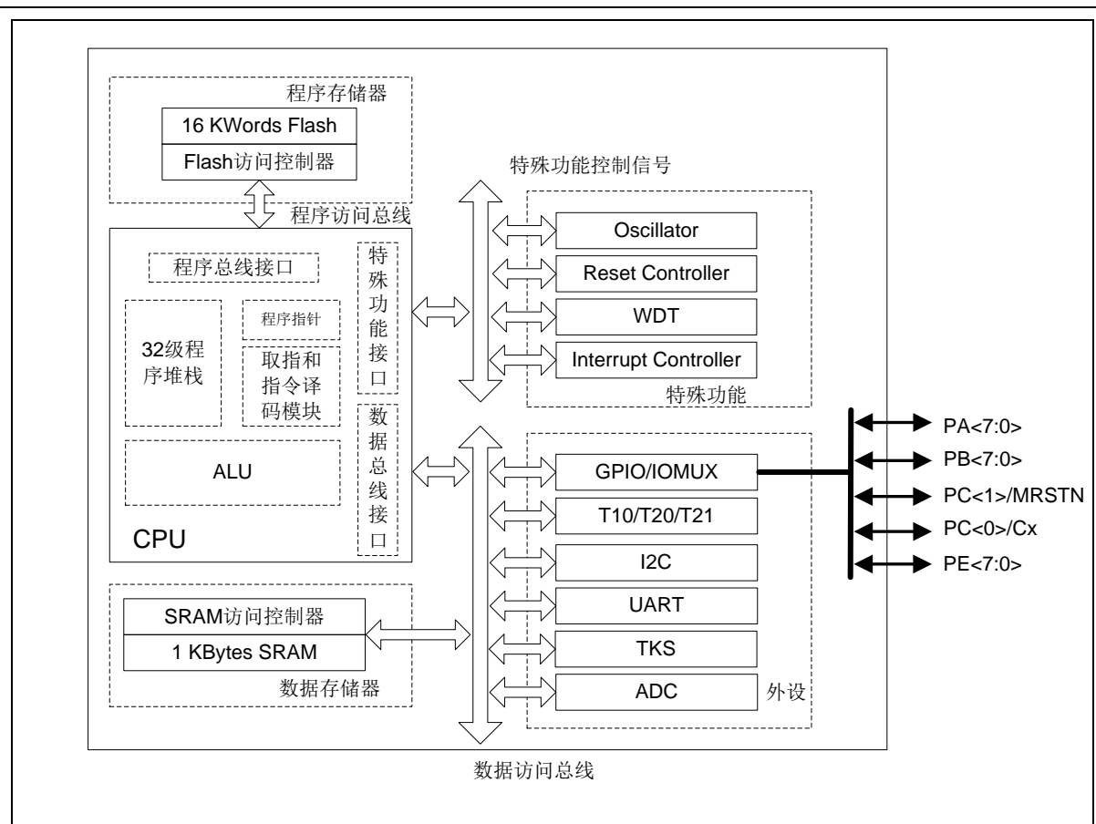
图 1-1 结构框图
