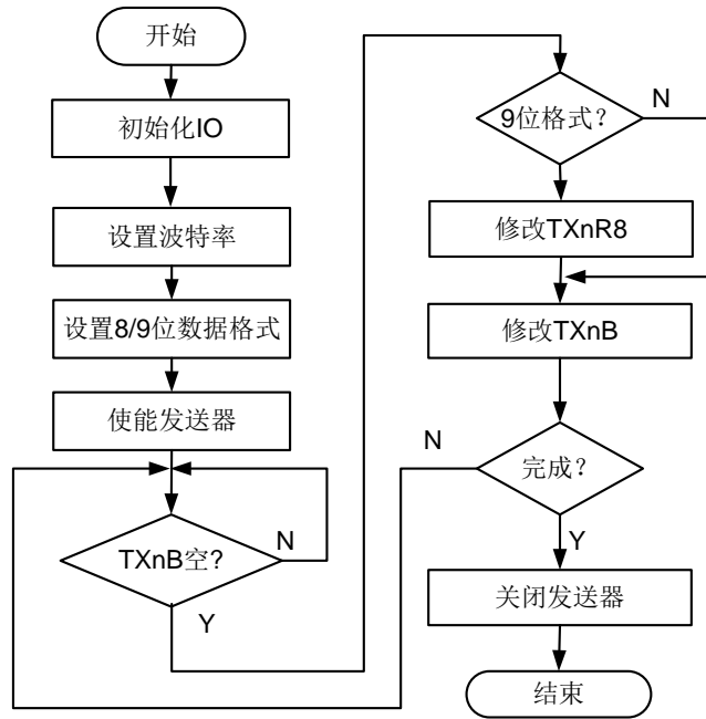
图 6-10 UARTn 发送器操作流程图
