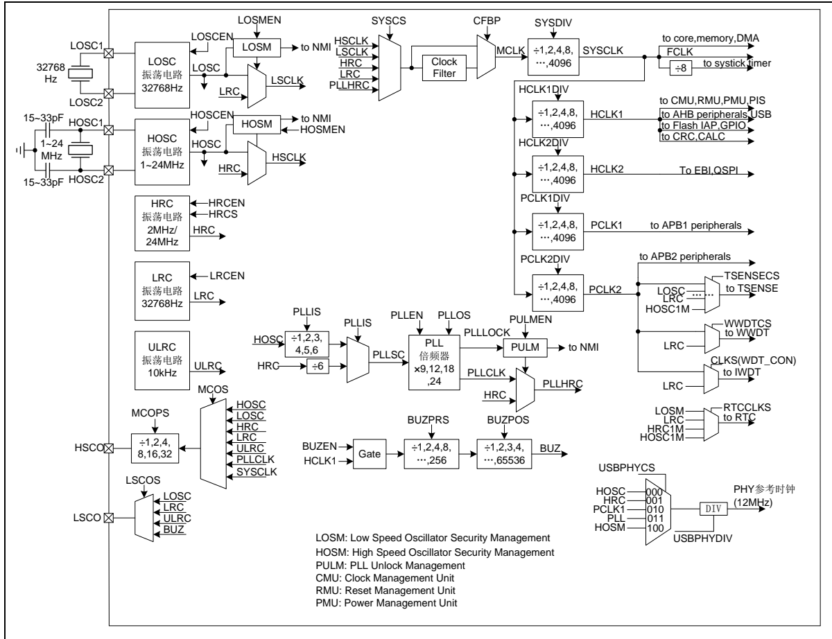
图 2-2 时钟树
