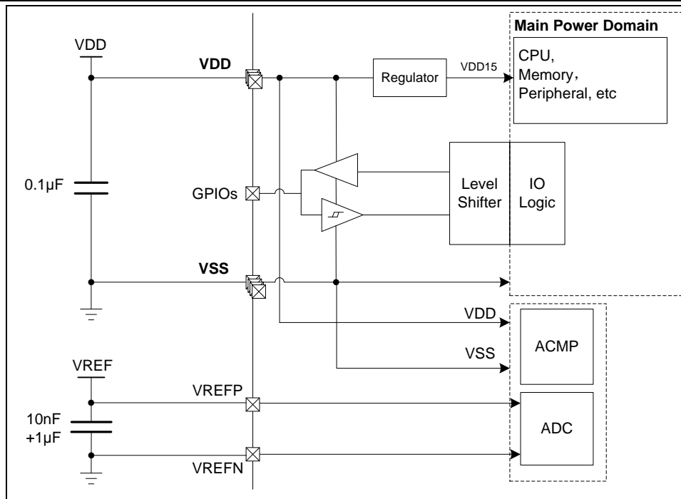
图 5-1 芯片电源
