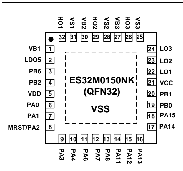
图 3-1 ES32M0150NKQFN32 顶视图
