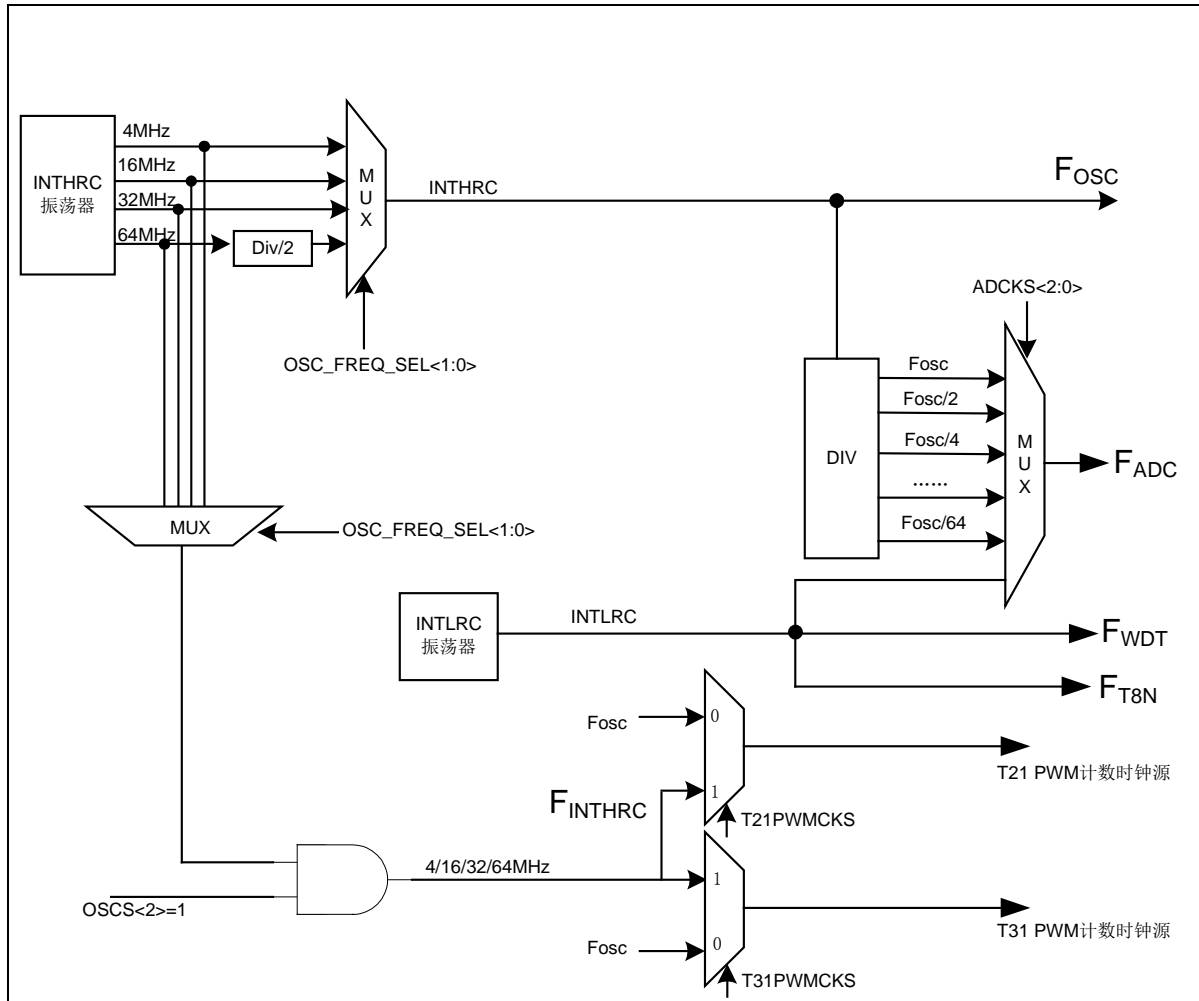
图 5-1 系统时钟结构图
