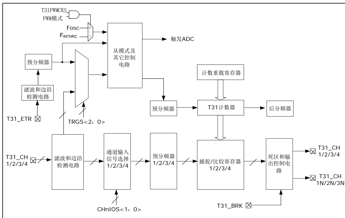
图 6-12 T31 内部结构图
