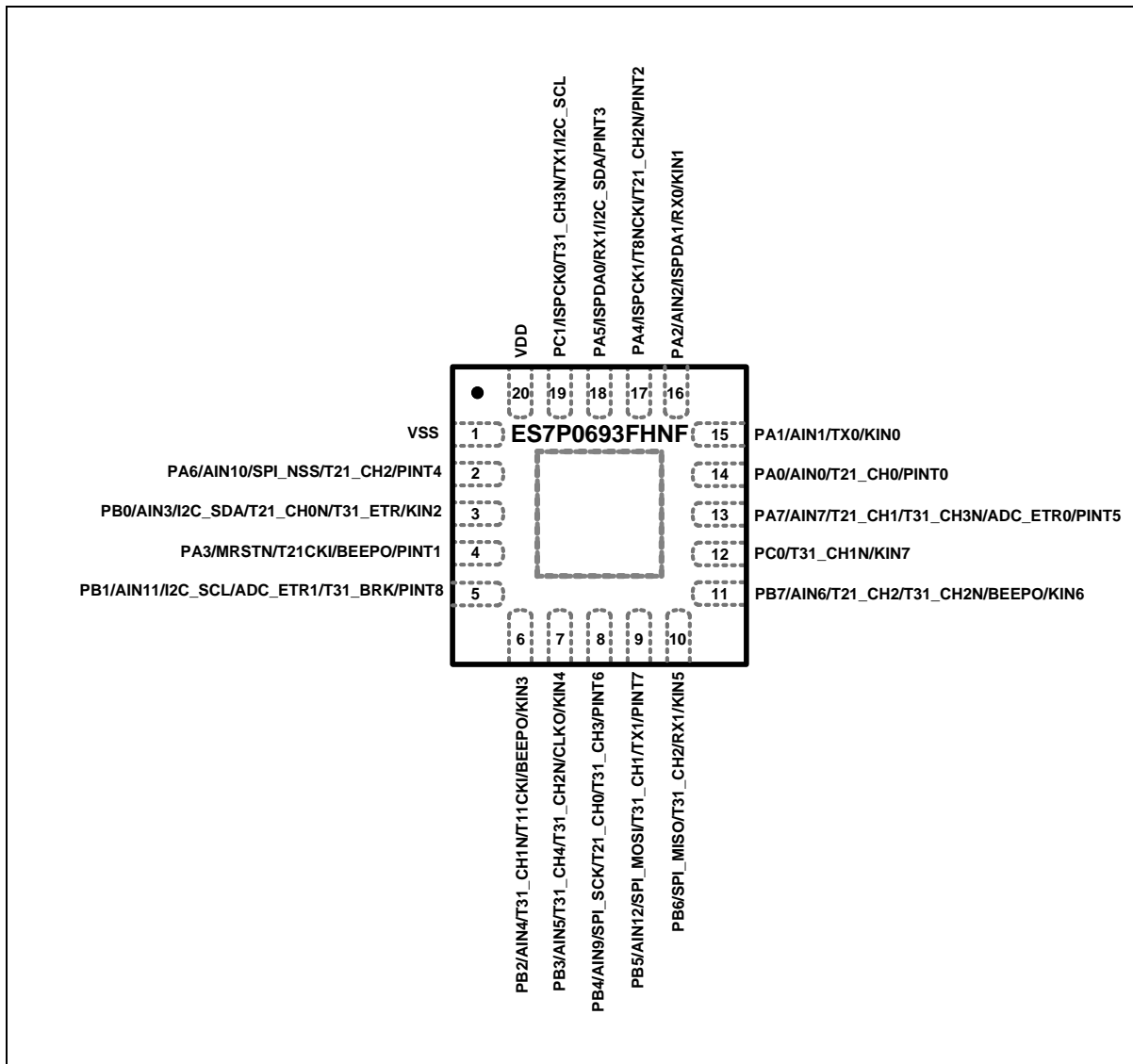
图 1-3 ES7P0693FHNQ 顶视图
