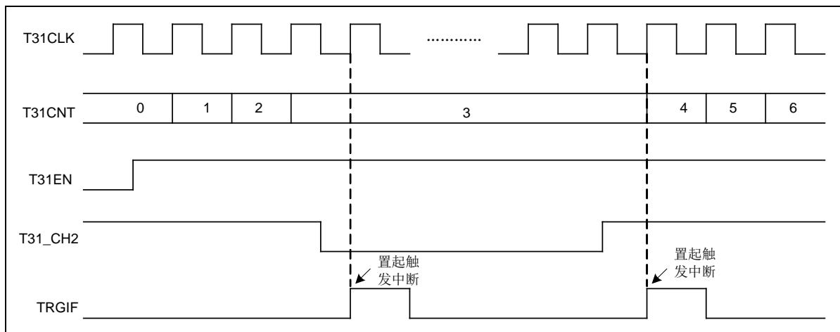
图 6-33 门控模式下的计数时序 (T31CNTLD=0x3F, 通道 2 端口门控信号高电平有效)
