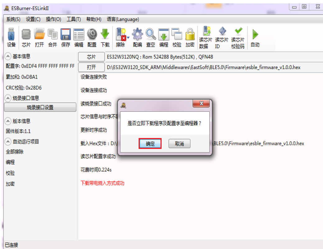
图 2-13 下载程序及配置字至编程器
