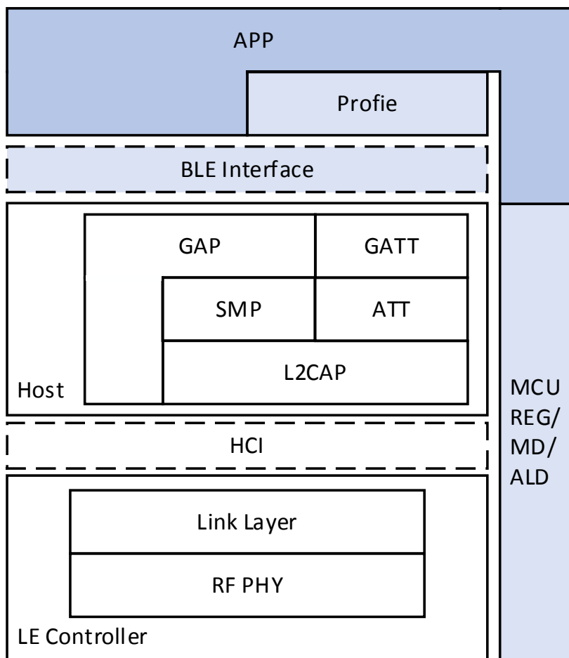
图 2-1 SDK 架构
