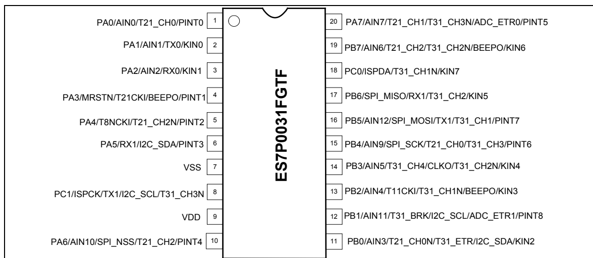
图 1-2 ES7P0031FGTF 顶视图
