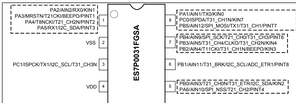
图 1-3 ES7P0031FGSA 顶视图
